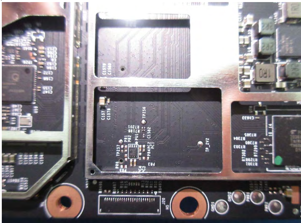
(40) EUT Photo
