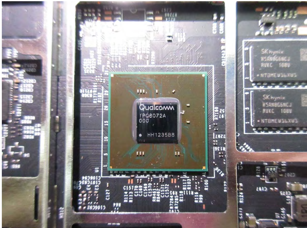
(40) EUT Photo
