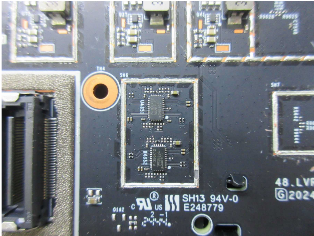
(100) EUT Photo
