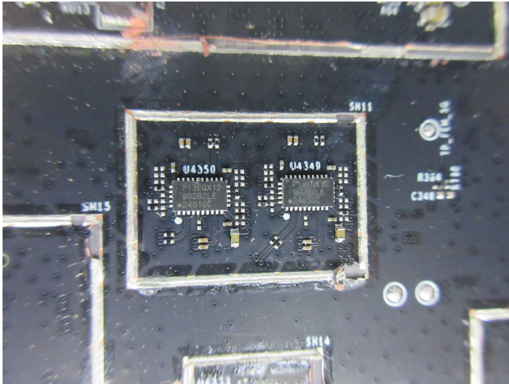
(86) EUT Photo
