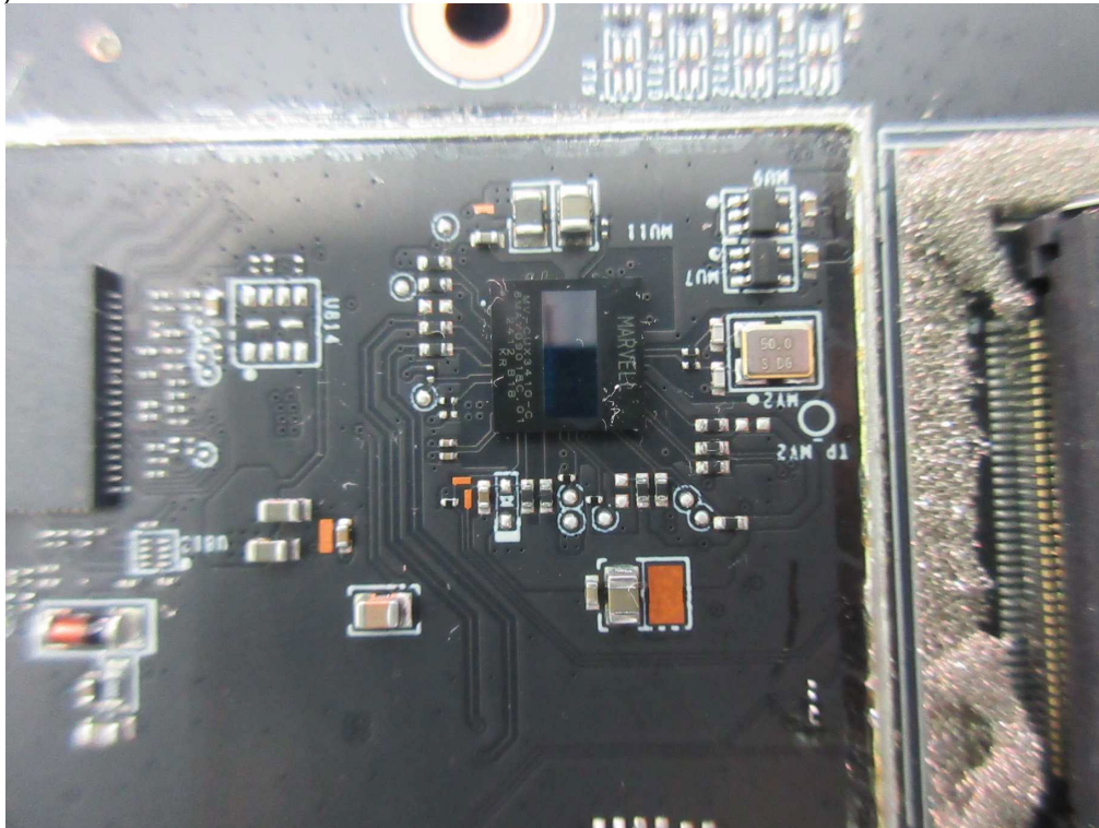
(106)EUT Photo
