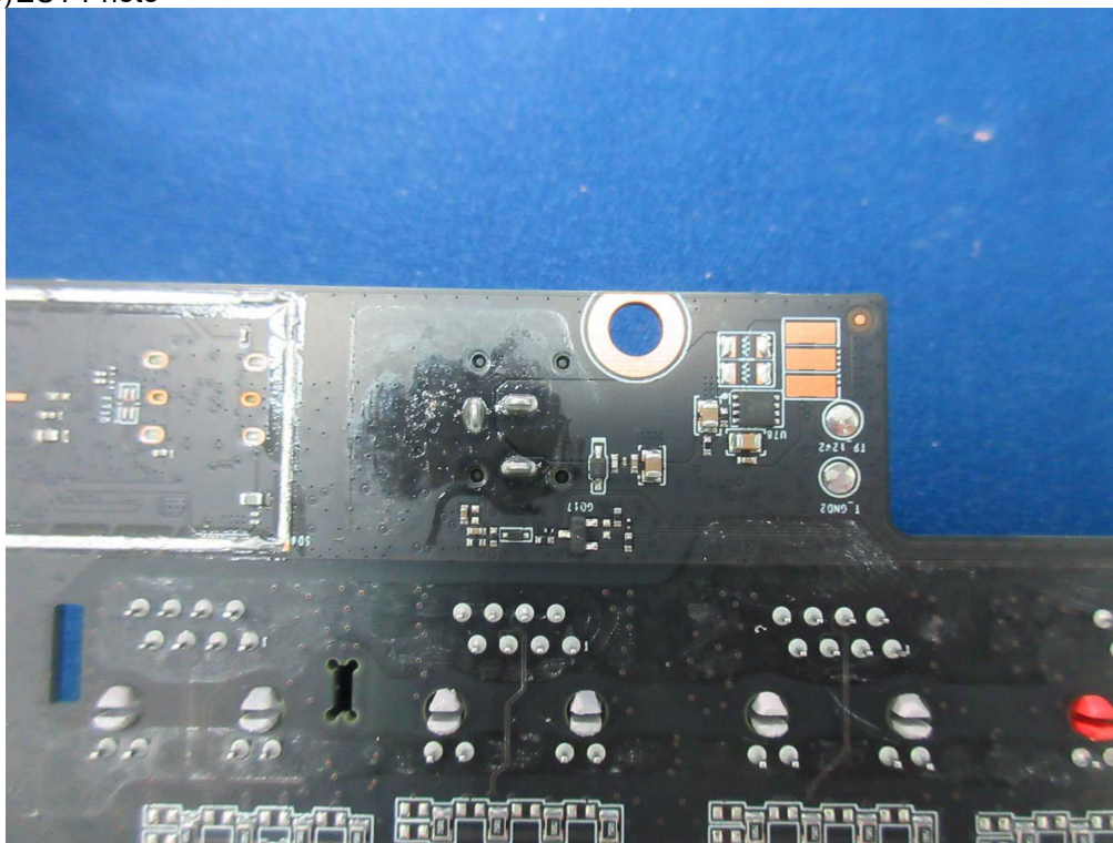
(108)EUT Photo
