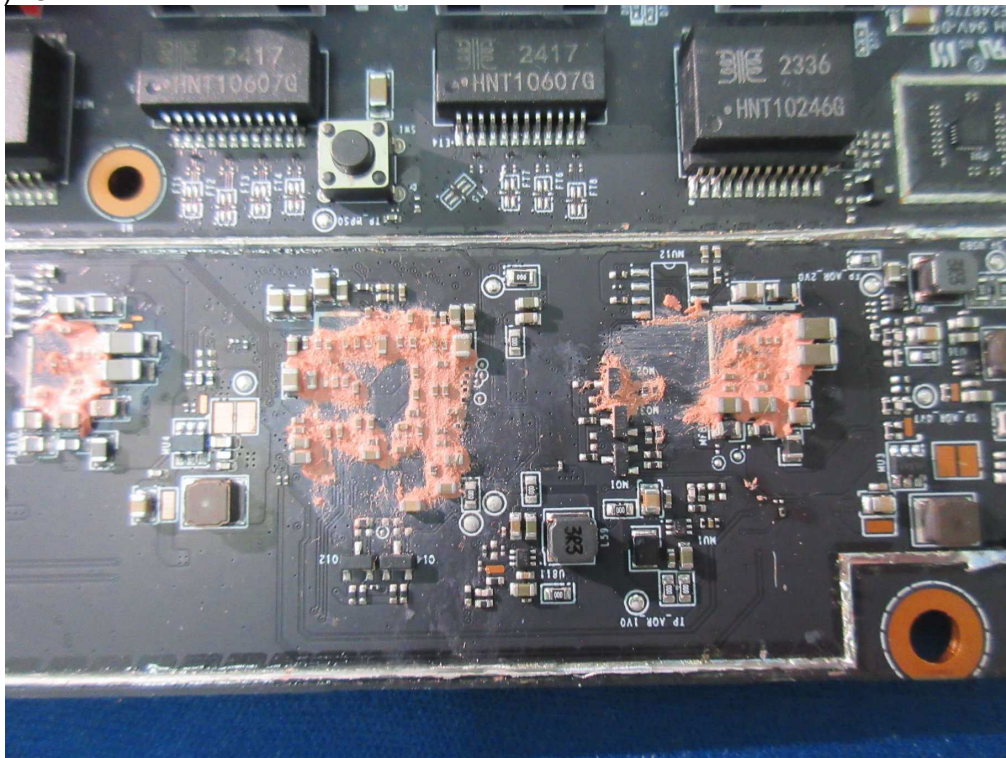
(118)EUT Photo
