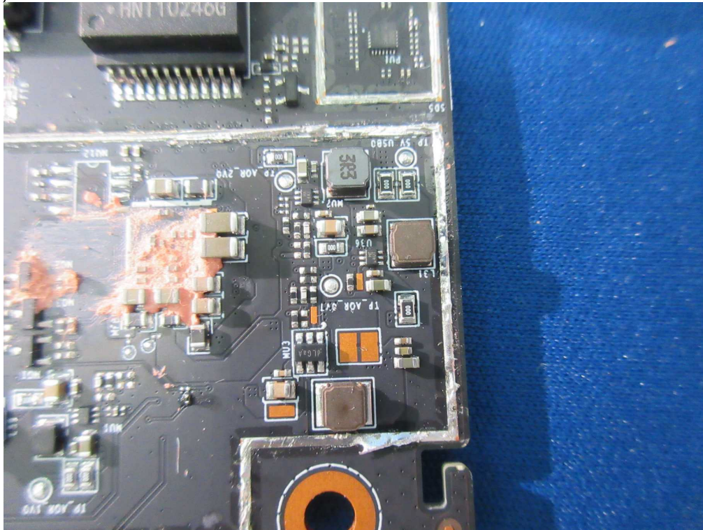
(120)EUT Photo
