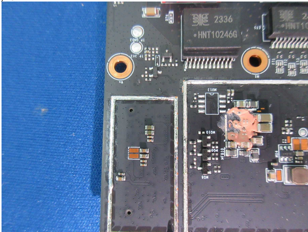
(116)EUT Photo
