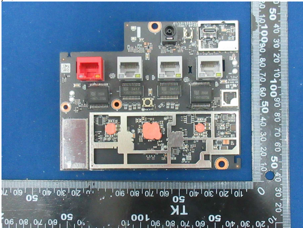
(110)EUT Photo
