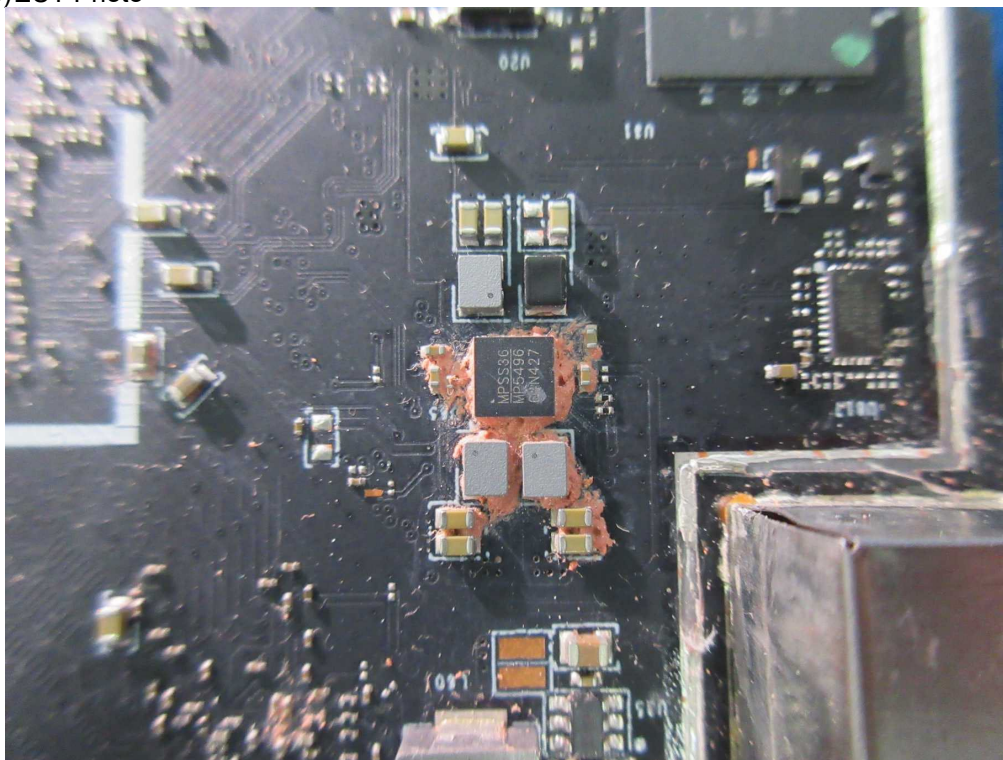
(136)EUT Photo
