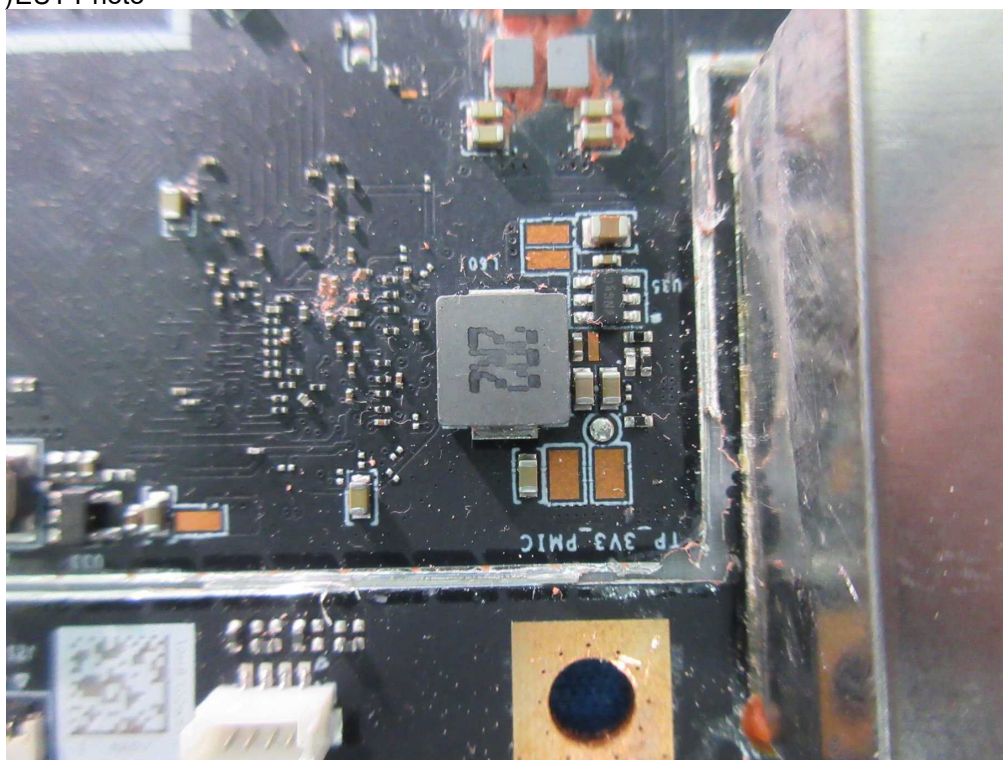
(137)EUT Photo
