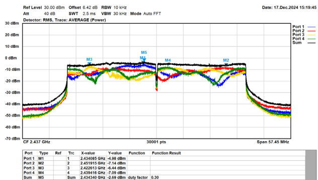
802.11be/40MHz/MCS0/2437MHz/Ch6
