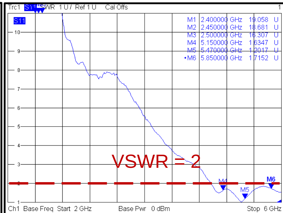
Ant. 1
