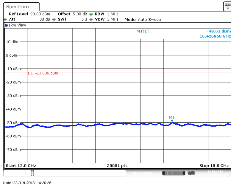
BAND 12_10MHz_QPSK_23130_1RB#0
