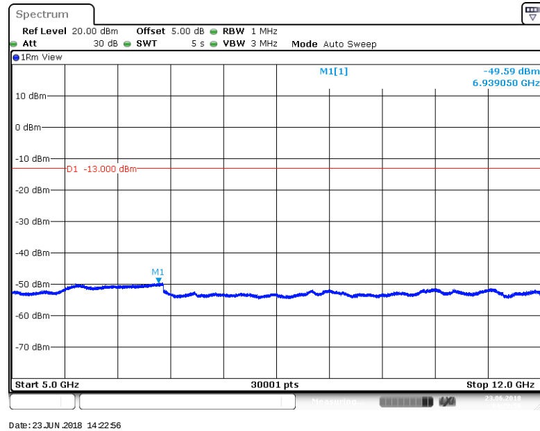
BAND 12_10MHz_QPSK_23130_1RB#0
