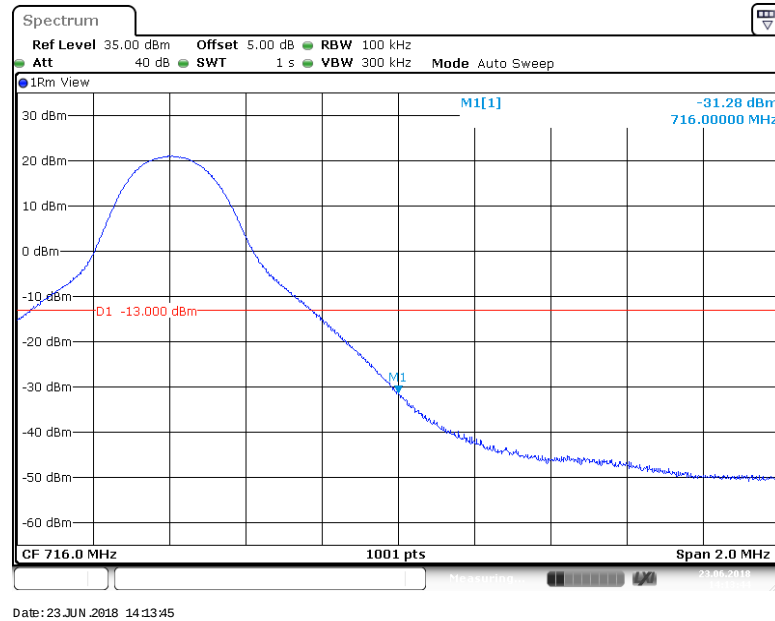
BAND 12_10MHz_QPSK_23130_50RB#0
