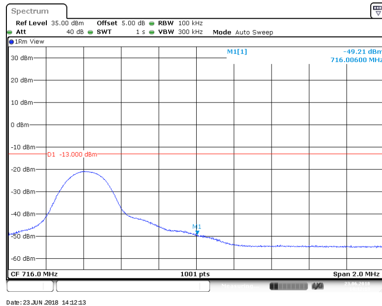
BAND 12_10MHz_QPSK_23130_1RB#49
