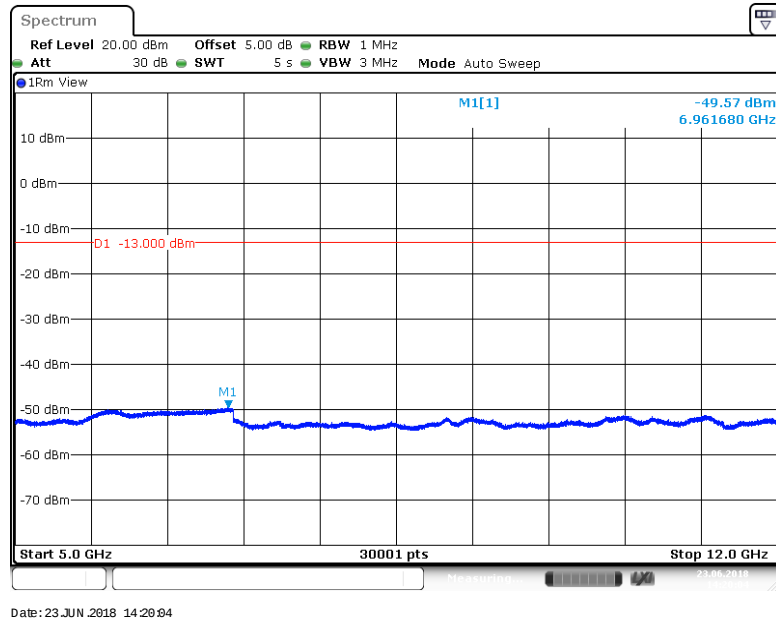
BAND 12_10MHz_QPSK_23095_1RB#0
