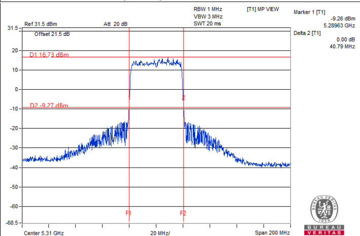
802.11ax (HE40) Beamforming / Chain1 : CH 62
