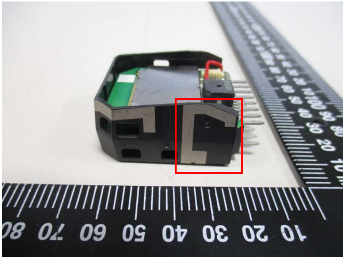
GPS antenna
