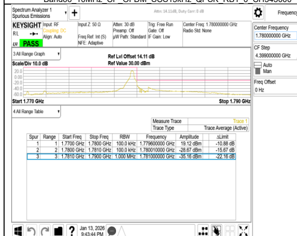
Band66 10MHz CP OFDM SCS15kHz QPSK RB1_51 CH355000
