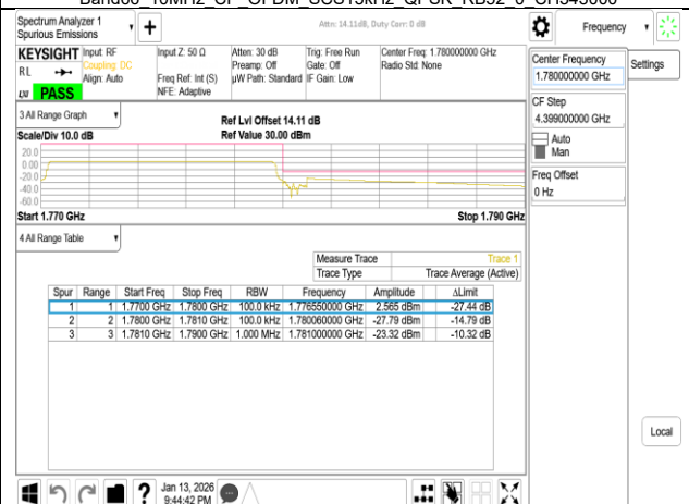
Band66 10MHz CP OFDM SCS15kHz QPSK RB52_0 CH355000
