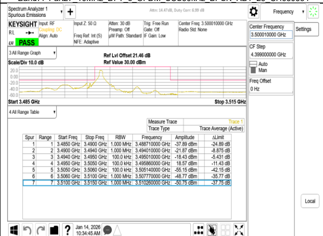
Band77-Part27 10MHz DFT s OFDM SCS30kHz BPSK RB1_0 CH633334
