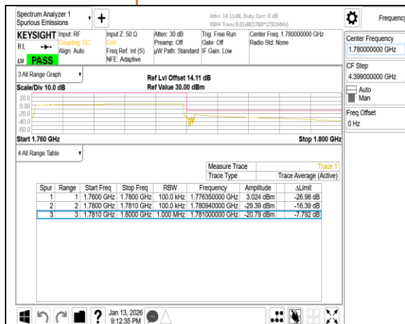
Band66 20MHz CP OFDM SCS15kHz QPSK RB106_0 CH354000
