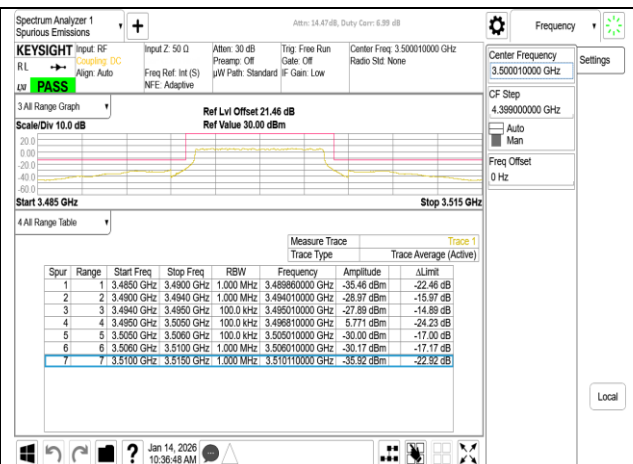
Band77-Part27 10MHz DFT s OFDM SCS30kHz BPSK RB24 0 CH633334
