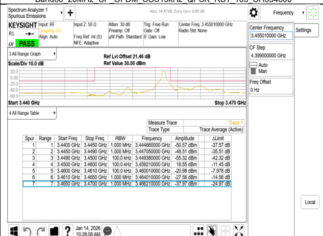
Band77-Part27 10MHz DFT s OFDM SCS30kHz BPSK RB1_23 CH630334
