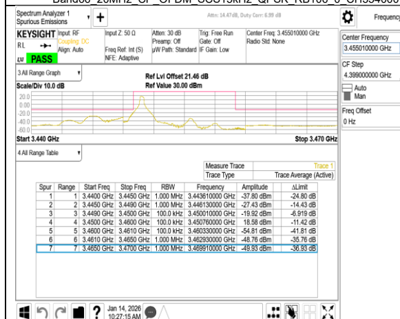
Band77-Part27 10MHz DFT s OFDM SCS30kHz BPSK RB1_0 CH630334
