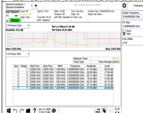
Band77-Part27 10MHz CP OFDM SCS30kHz QPSK RB1 0 CH656000
