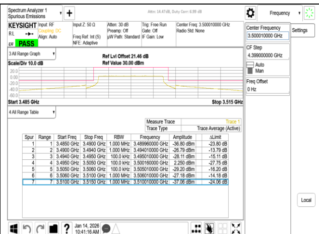
Band77-Part27 10MHz CP OFDM SCS30kHz QPSK RB24 0 CH633334
