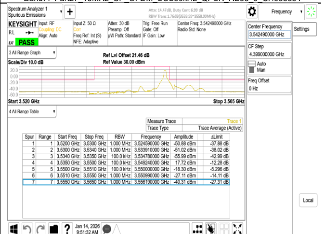
Band77-Part27 15MHz CP OFDM SCS30kHz QPSK RB1 37 CH636166
