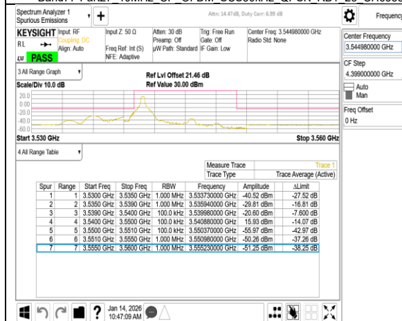
Band77-Part27 10MHz CP OFDM SCS30kHz QPSK RB1 0 CH636332
