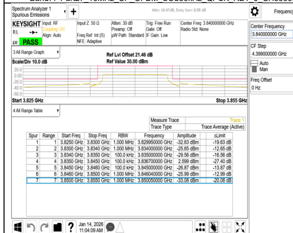
Band77-Part27 10MHz CP OFDM SCS30kHz QPSK RB24 0 CH656000
