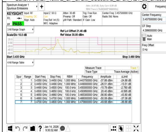
Band77-Part27 15MHz DFT s OFDM SCS30kHz BPSK RB1_0 CH630500
