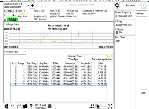
Band77-Part27 10MHz CP OFDM SCS30kHz QPSK RB1 0 CH647000
