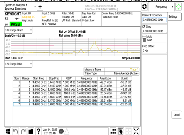
Band77-Part27 15MHz DFT s OFDM SCS30kHz BPSK RB1 37 CH630500
