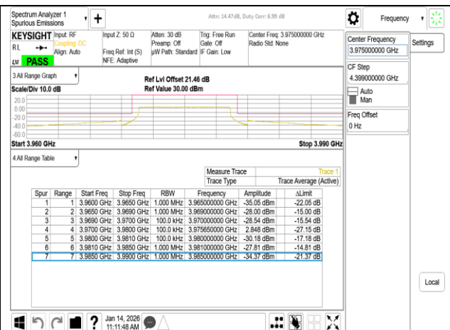
Band77-Part27 10MHz CP OFDM SCS30kHz QPSK RB24_0 CH665000
