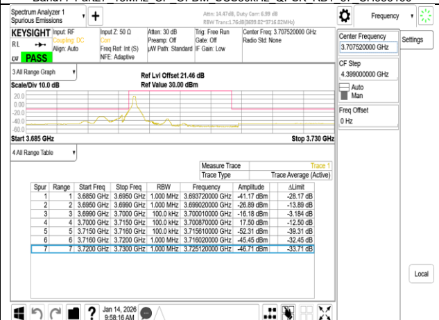
Band77-Part27 15MHz CP OFDM SCS30kHz QPSK RB1 0 CH647168
