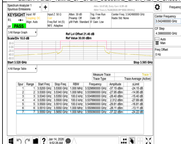
Band77-Part27 15MHz CP OFDM SCS30kHz QPSK RB38 0 CH636166
