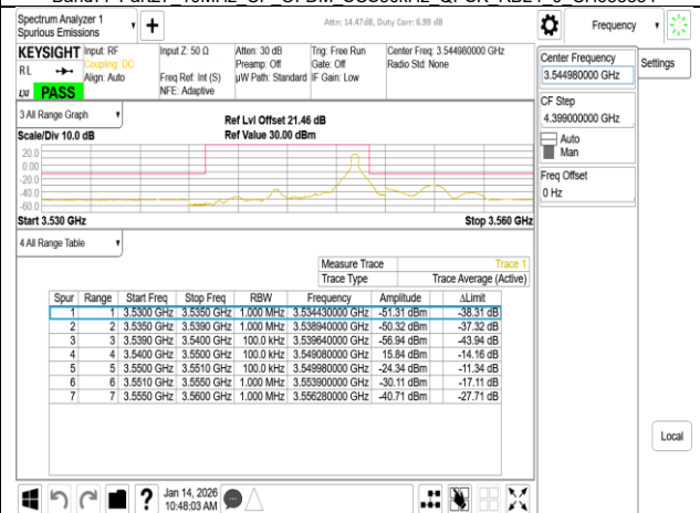
Band77-Part27 10MHz CP OFDM SCS30kHz QPSK RB1 23 CH636332
