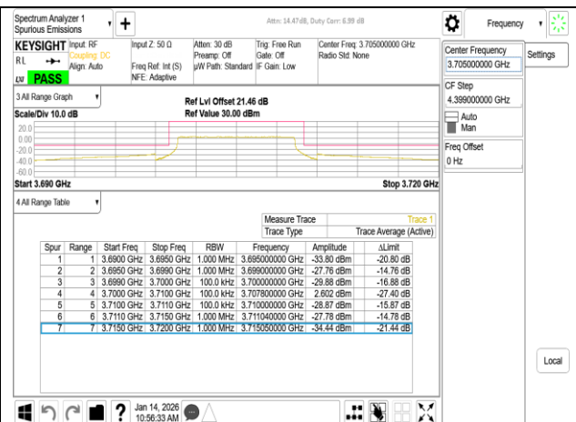
Band77-Part27 10MHz CP OFDM SCS30kHz QPSK RB24 0 CH647000
