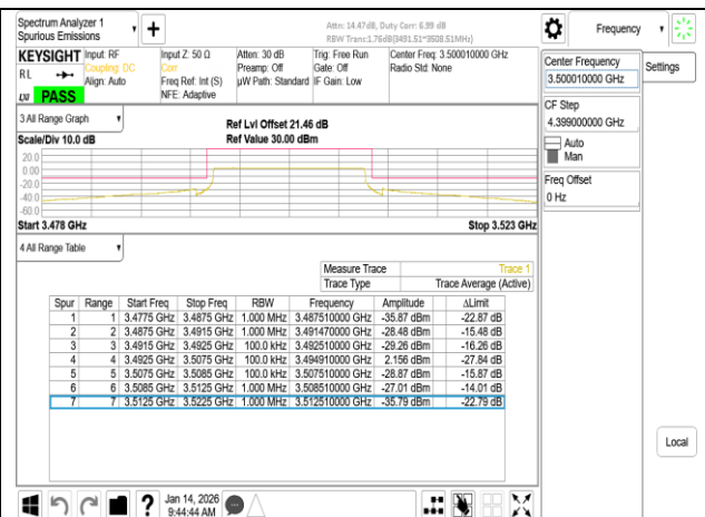
Band77-Part27 15MHz CP OFDM SCS30kHz QPSK RB38 0 CH633334
