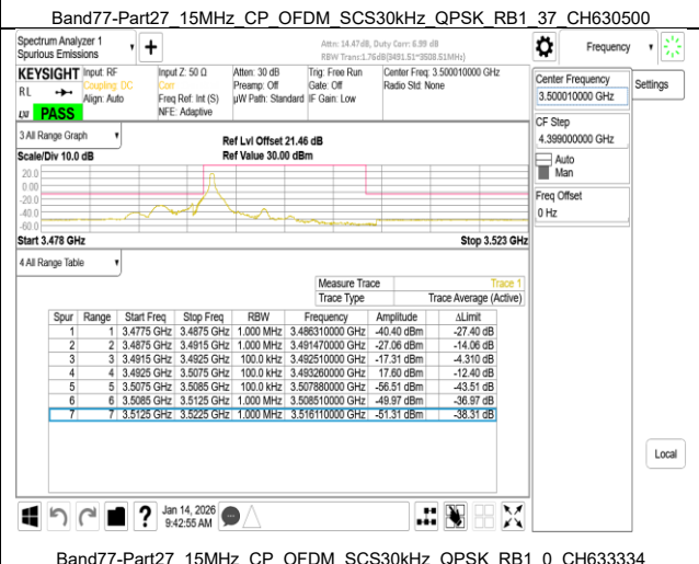
Band77-Part27 15MHz CP OFDM SCS30kHz QPSK RB1_0 CH633334
