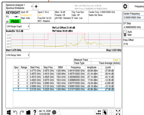
Band77-Part27 15MHz CP OFDM SCS30kHz QPSK RB1 37 CH633334
