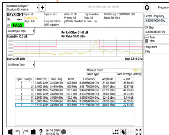
Band77-Part27 10MHz CP OFDM SCS30kHz QPSK RB1 23 CH633334
