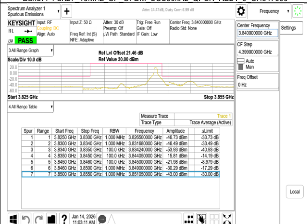
Band77-Part27 10MHz CP OFDM SCS30kHz QPSK RB1 23 CH656000
