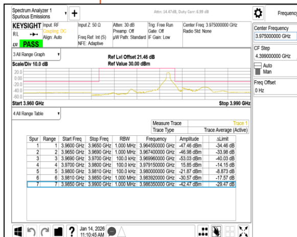
Band77-Part27 10MHz CP OFDM SCS30kHz QPSK RB1 23 CH665000
