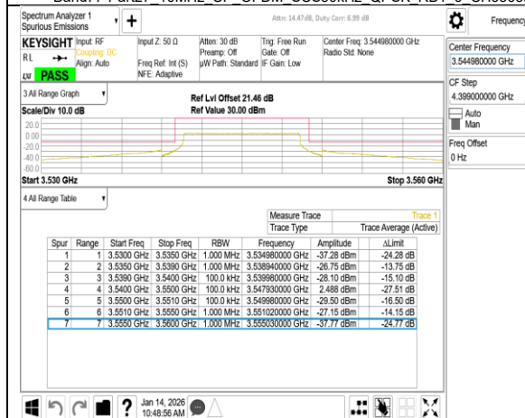
Band77-Part27 10MHz CP OFDM SCS30kHz QPSK RB24 0 CH636332
