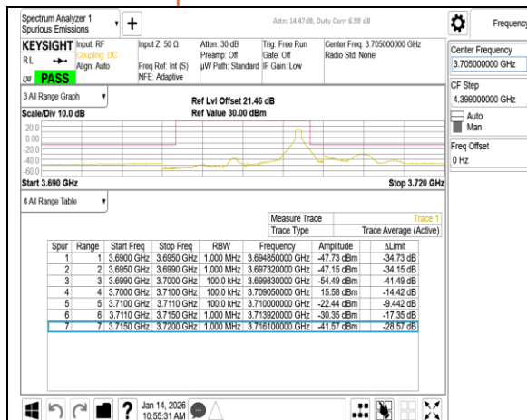
Band77-Part27 10MHz CP OFDM SCS30kHz QPSK RB1 23 CH647000
