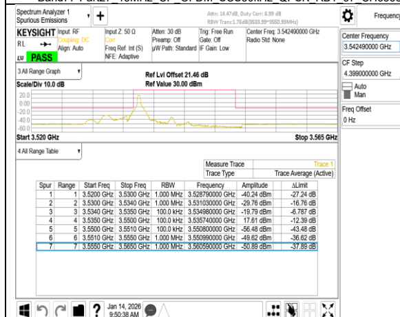
Band77-Part27 15MHz CP OFDM SCS30kHz QPSK RB1 0 CH636166
