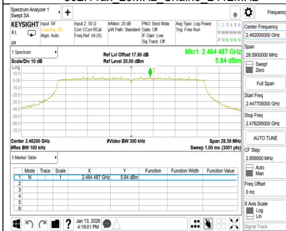
802.11ax 20MHz Chain0 2462MHz
