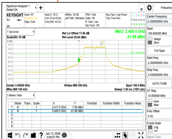
802.11g 20MHz Chain1 2412MHz
