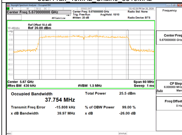
802.11ax 40MHz Chain0 5670MHz
