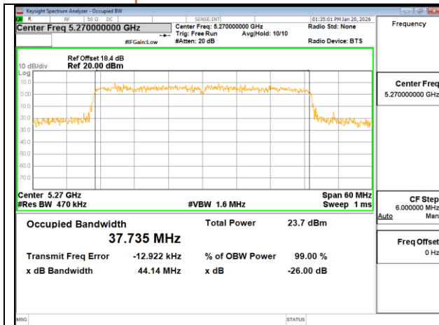
802.11ax 40MHz Chain0 5270MHz
