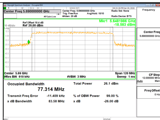
802.11ax 80MHz Chain1 5690MHz UNII-2C
