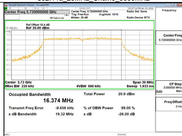
802.11a 20MHz Chain0 5720MHz
