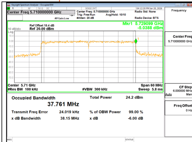
802.11ax 40MHz Chain0 5710MHz UNII-3
