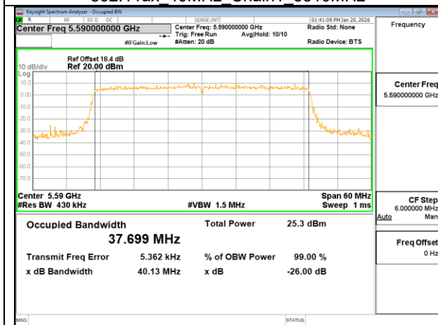
802.11ax 40MHz Chain1 5590MHz
