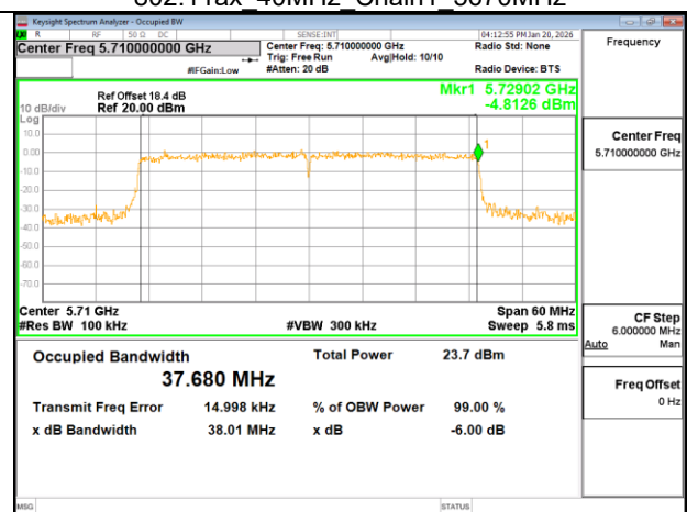
802.11ax 40MHz Chain1 5710MHz UNII-3
