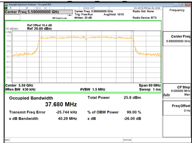
802.11ax 40MHz Chain0 5590MHz
