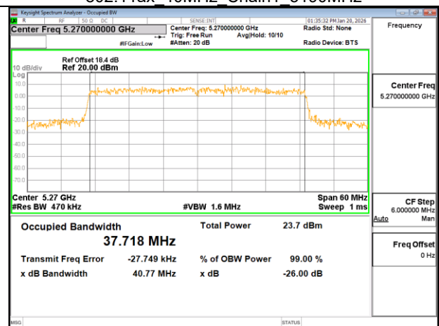
802.11ax 40MHz Chain1 5270MHz
