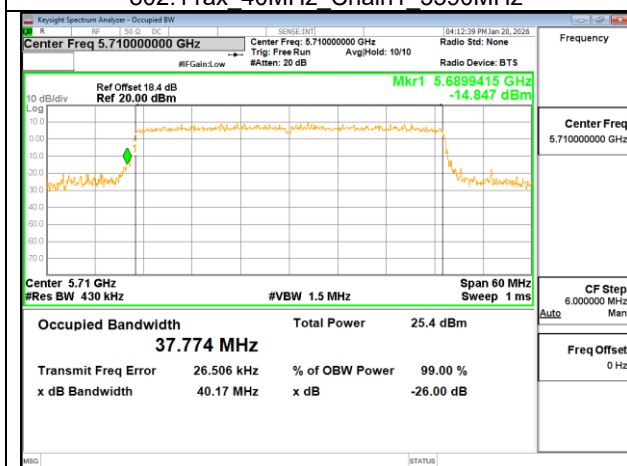
802.11ax 40MHz Chain1 5710MHz UNII-2C
