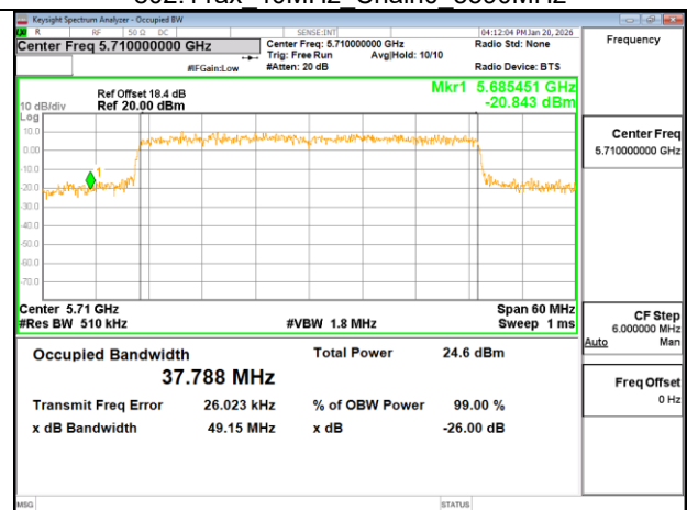
802.11ax 40MHz Chain0 5710MHz_UNII-2C
