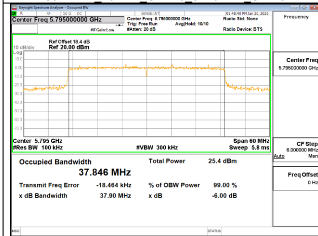
802.11ax 40MHz Chain0 5795MHz
