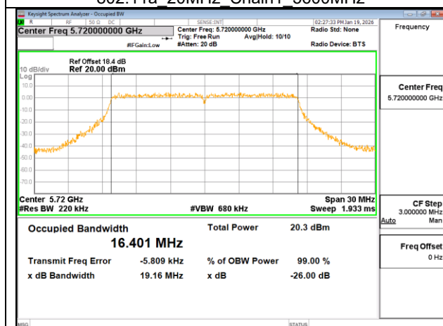
802.11a 20MHz Chain1 5720MHz
