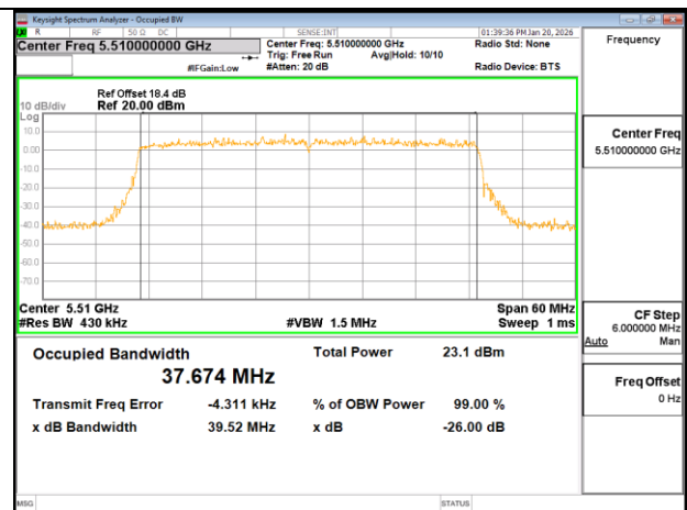
802.11ax 40MHz Chain1 5510MHz
