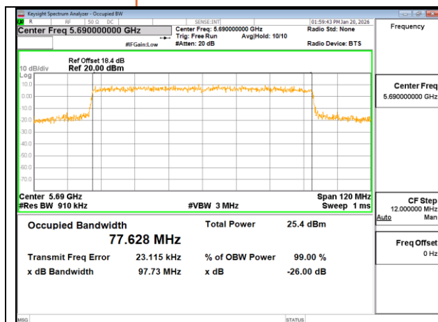
802.11ax 80MHz Chain0 5690MHz
