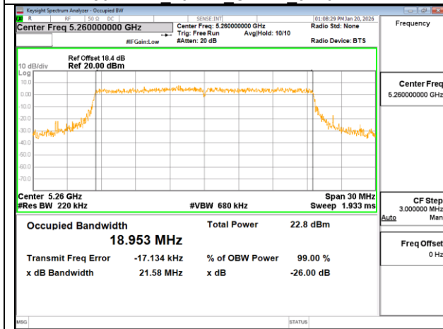
802.11ax 20MHz Chain1 5260MHz
