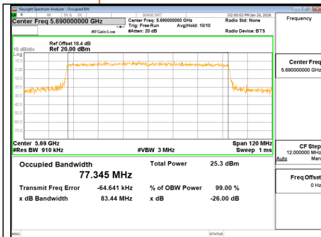
802.11ax 80MHz Chain1 5690MHz
