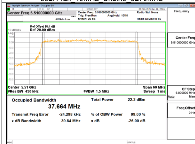
802.11ax 40MHz Chain0 5510MHz
