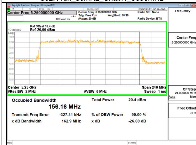
802.11ax 160MHz Chain0 5250MHz
