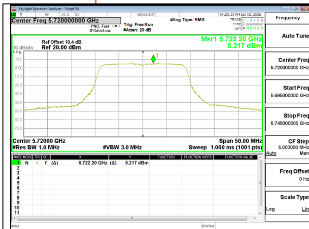
802.11n 20MHz Chain1 5720MHz UNII 2C
