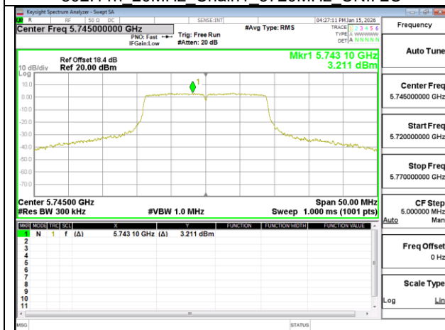
802.11n 20MHz Chain0 5745MHz
