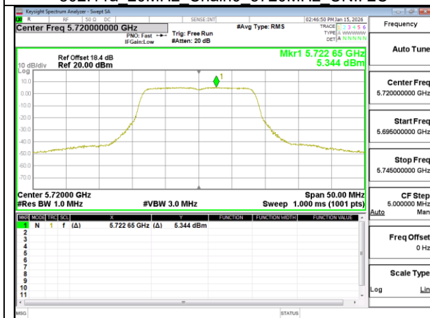
802.11a 20MHz Chain1 5720MHz UNII 2C
