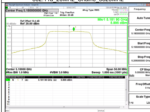
802.11n 20MHz Chain0 5180MHz
