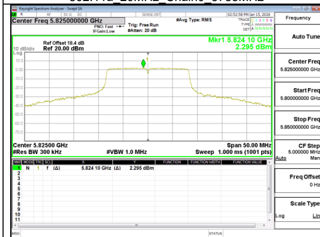
802.11a 20MHz Chain0 5825MHz
