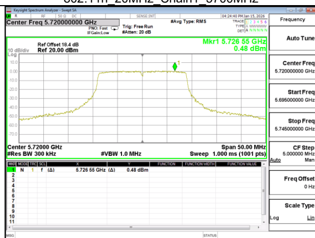
802.11n 20MHz Chain0 5720MHz UNII 3
