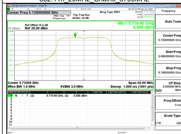
802.11n 20MHz Chain0 5720MHz UNII 2C
