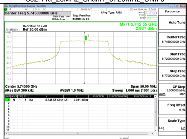
802.11a 20MHz Chain1 5745MHz
