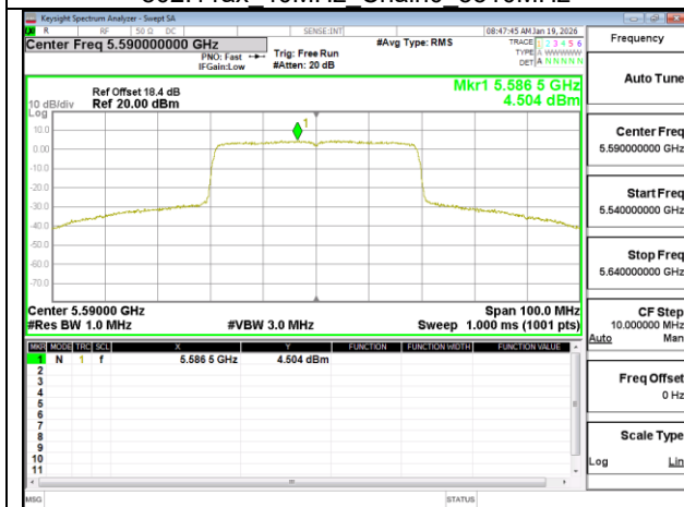
802.11ax 40MHz Chain0 5590MHz
