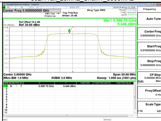
802.11ax 20MHz Chain1 5600MHz
