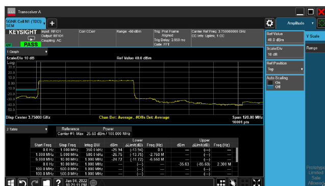
5G NR n77 CH 66366650M pi/2 BPSK 128RB5
