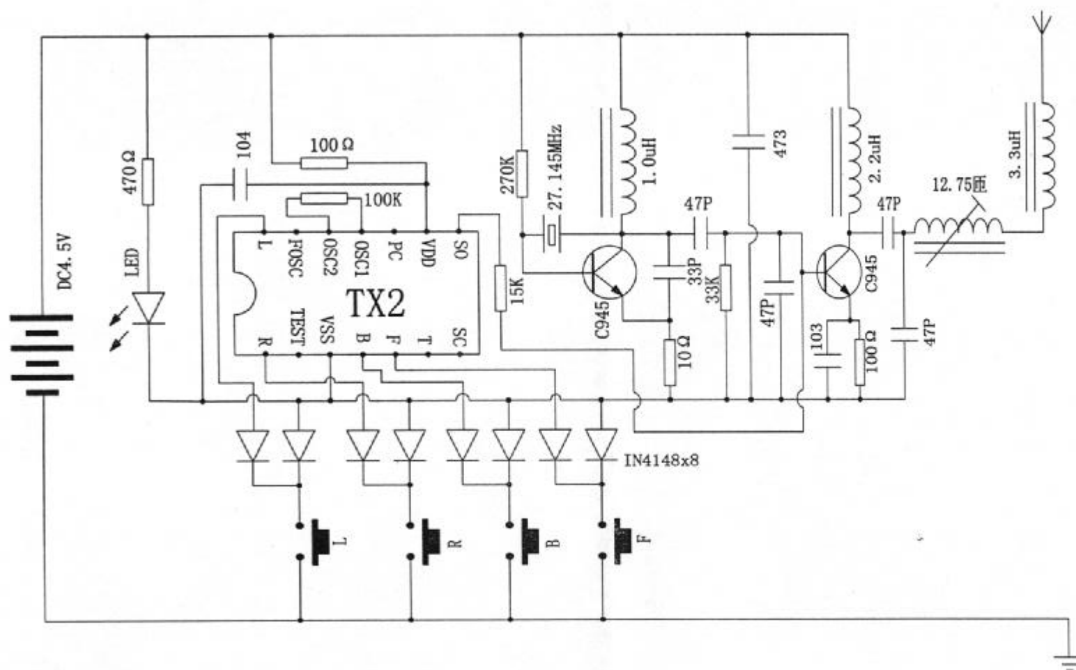
27MHz Q版车 (B888) 发射器原理图
