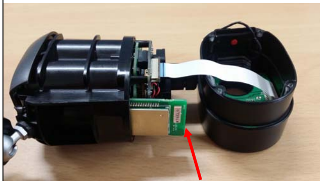
900MHz Antenna
