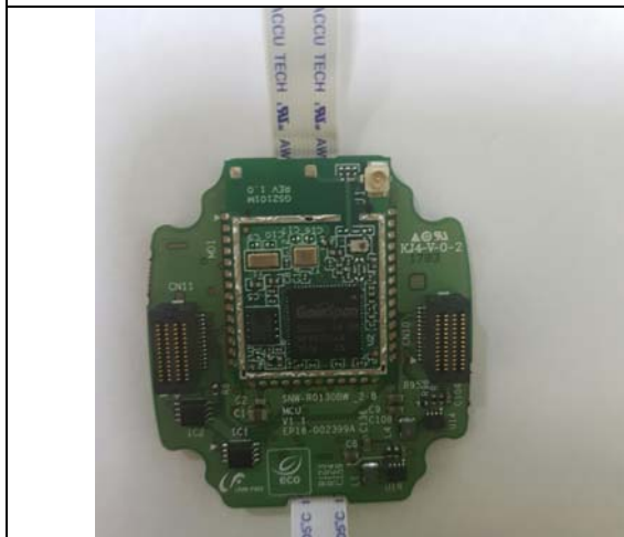
900MHz Antenna
