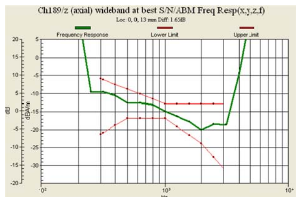
Fig 7.1 GSM850 Ch189
