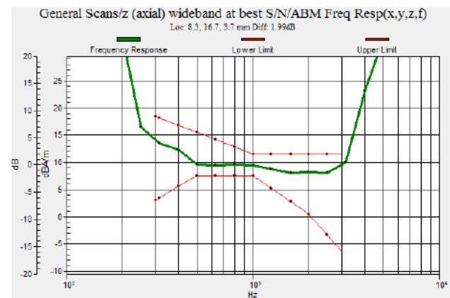
Fig. 7.6 CDMA BC 1
