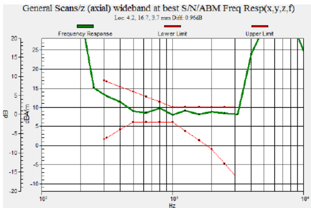
Fig. 7.5 CDMA BC 0
