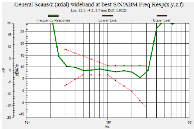
Fig 7.1 GSM850
