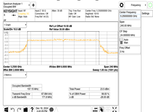
802.11ax_160MHz_Chain0_5250MHz
