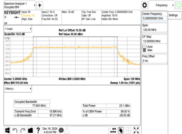
802.11ax_80MHz_Chain0_5290MHz
