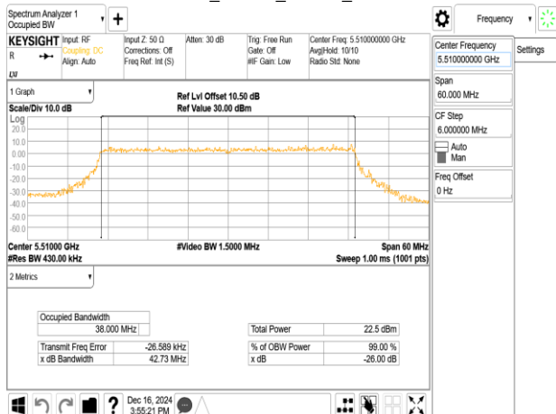
802.11ax_40MHz_Chain0_5510MHz
