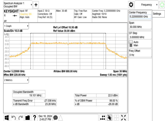
802.11ax_20MHz_Chain0_5220MHz
