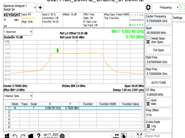
802.11ax_20MHz_Chain0_5700MHz_RU26_8
