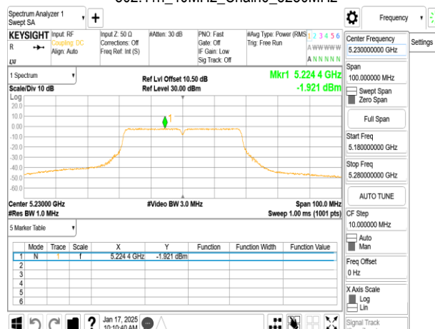
802.11n_40MHz_Chain0_5230MHz
