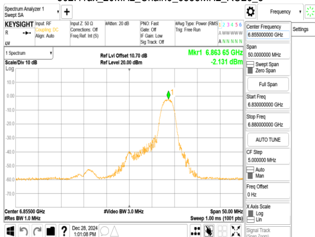
802.11ax_20MHz_Chain0_6855MHz_RU52_40
