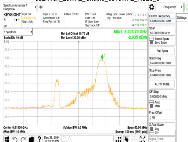
802.11ax_20MHz_Chain0_6515MHz_RU52_40
