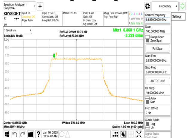
802.11ax_40MHz_Chain0_6885MHz
