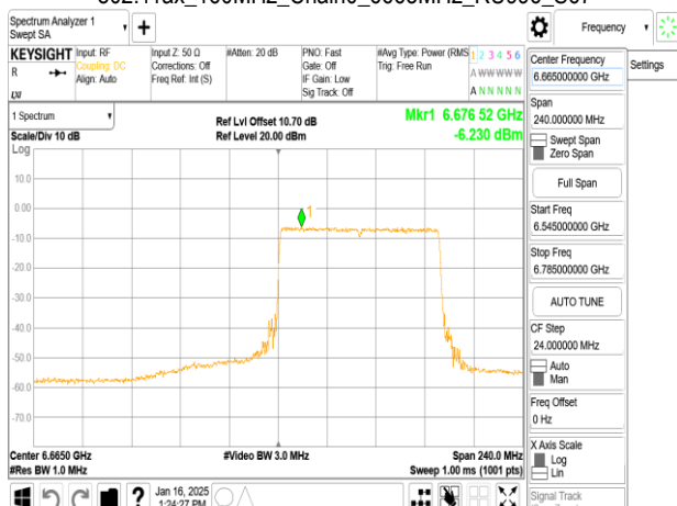
802.11ax_160MHz_Chain0_6665MHz_RU996_S67
