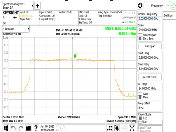
802.11ax_160MHz_Chain0_6025MHz_RU996_67
