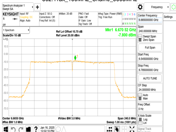
802.11ax_160MHz_Chain0_6665MHz_RU996_67
