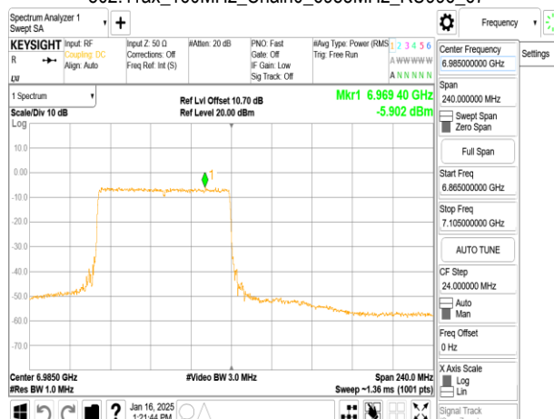
802.11ax_160MHz_Chain0_6985MHz_RU996_67
