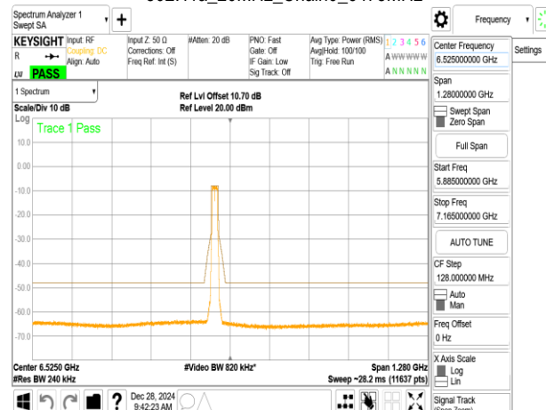
802.11a_20MHz_Chain0_6515MHz
