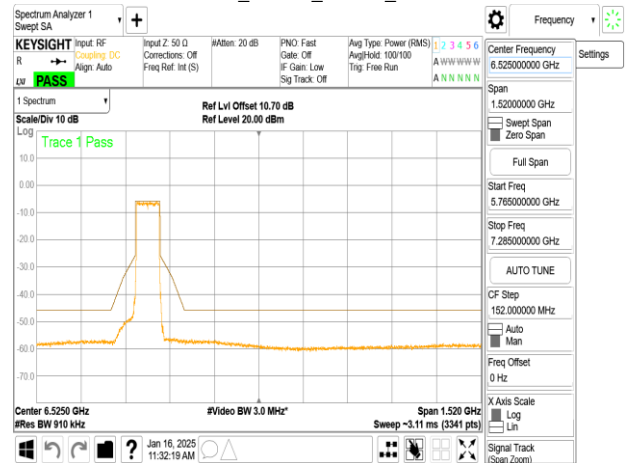
802.11ax_80MHz_Chain0_6385MHz
