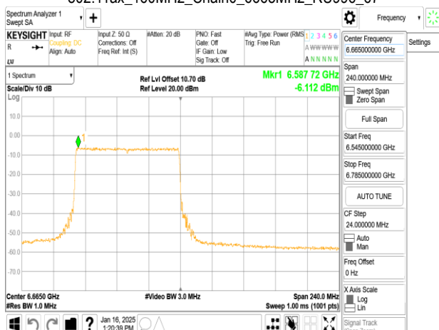
802.11ax_160MHz_Chain0_6665MHz_RU996_S67
