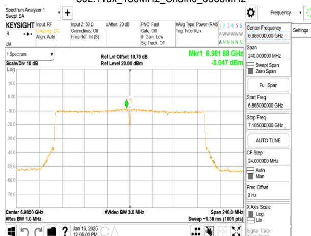
802.11ax_160MHz_Chain0_6985MHz_RU996_67
