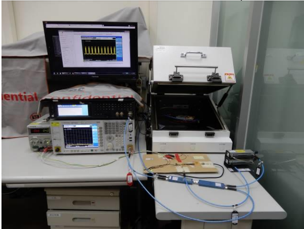
FCC_15_407_WLAN_6E_Normal_CBP_Setup
