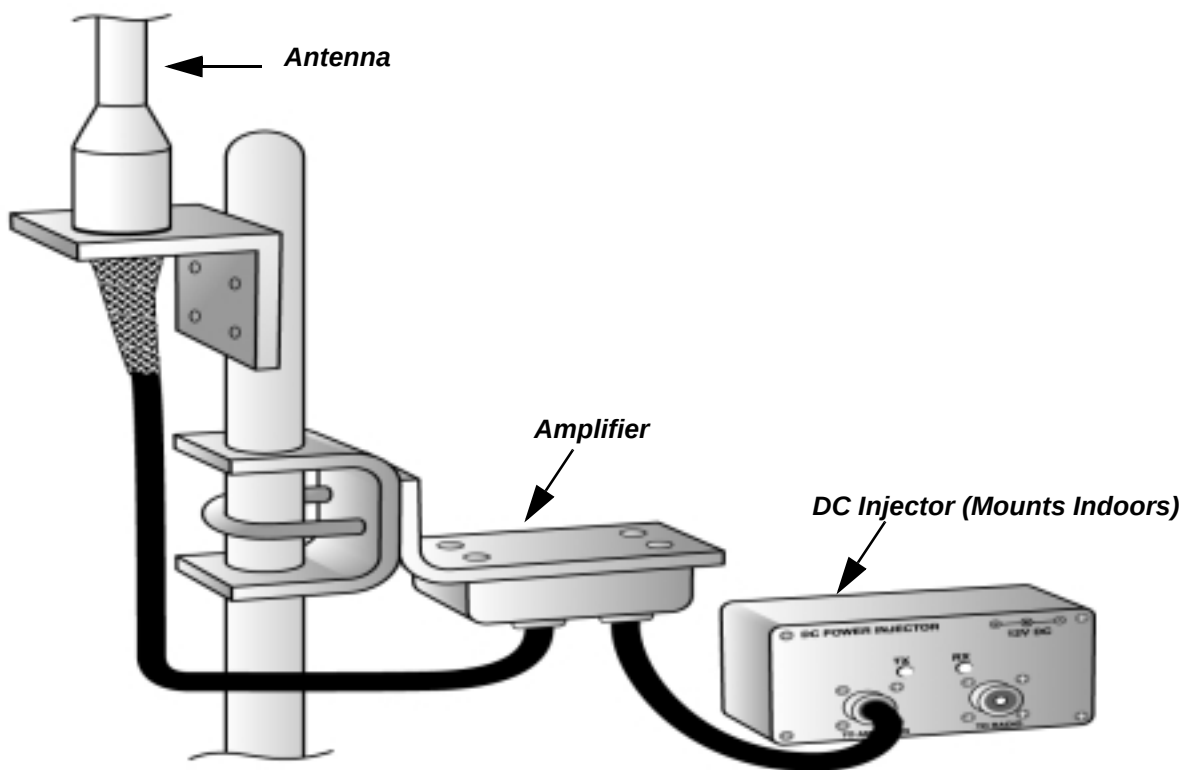
Amplifier Wiring
