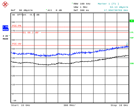
15 GHz – 18 GHz
