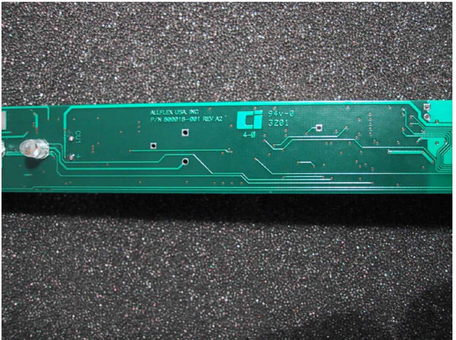
PCB BOTTOM B
