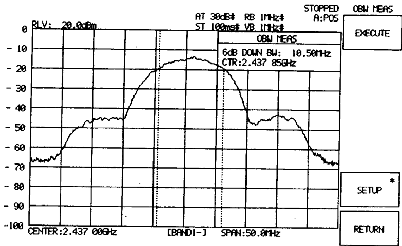
Fig CH6 (2437MHz)
