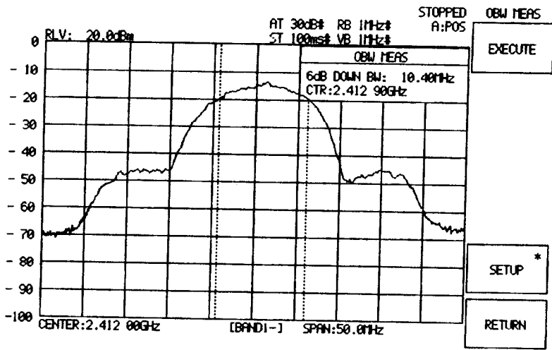
Fig CH1 (2412MHz)
