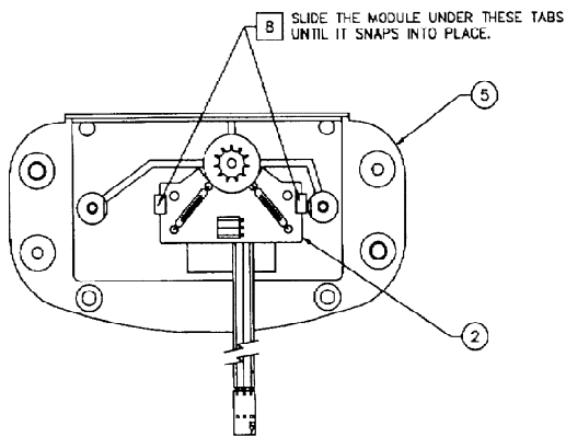
SENSOR MODULE SCALE: 1:1
