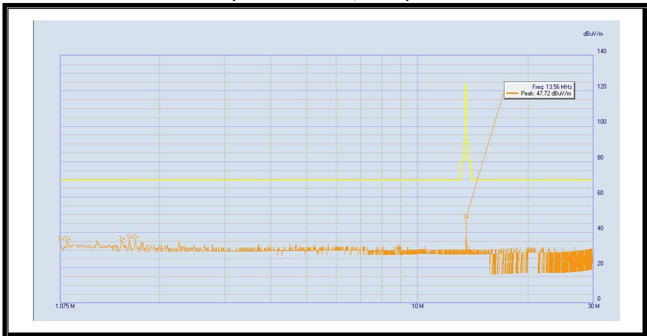
(Plot A: 1.075MHz – 30MHz)
