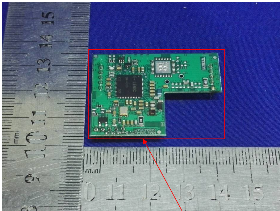
13.56MHz Module
