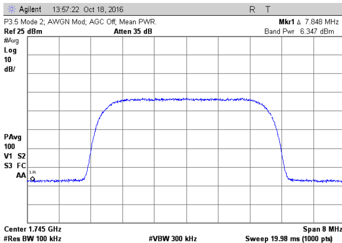
1745 MHz AWGN
