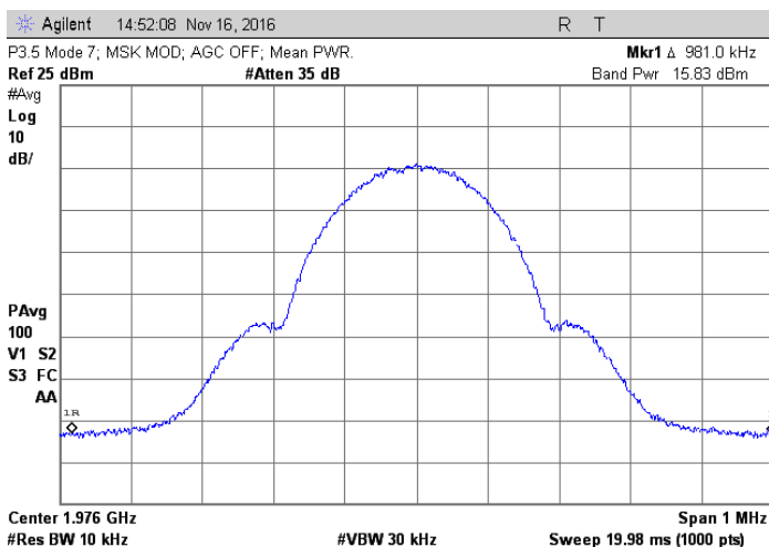
1976.2 MHz; MSK
