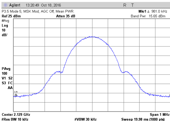
2129 MHz; MSK
