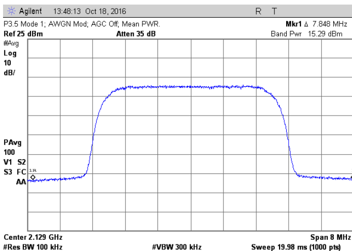
2129 MHz; AWGN
