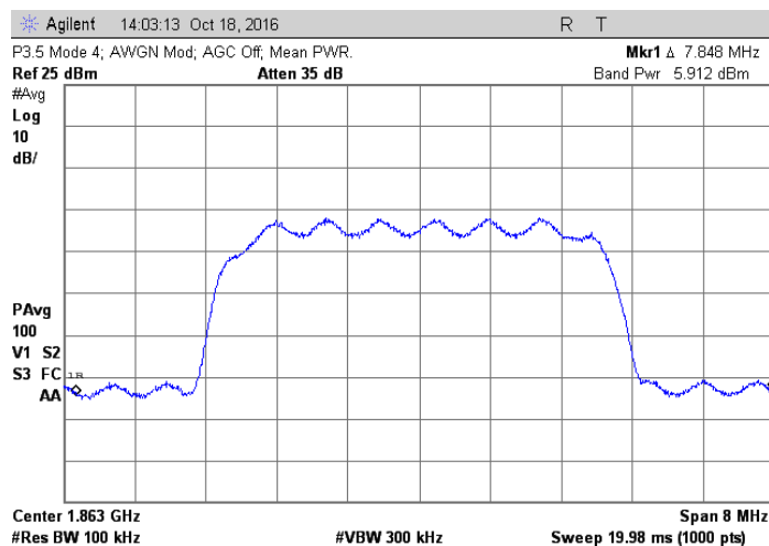
1863 MHz AWGN
