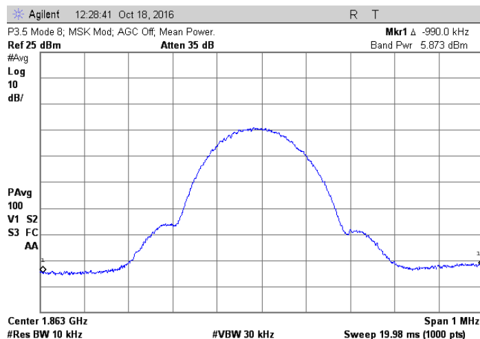
1863 MHz MSK
