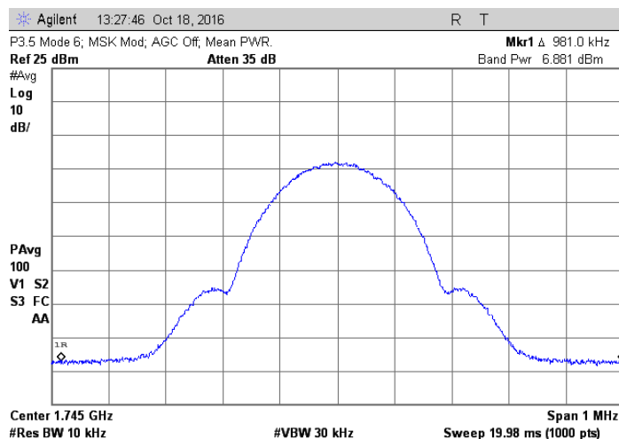
1745 MHz MSK
