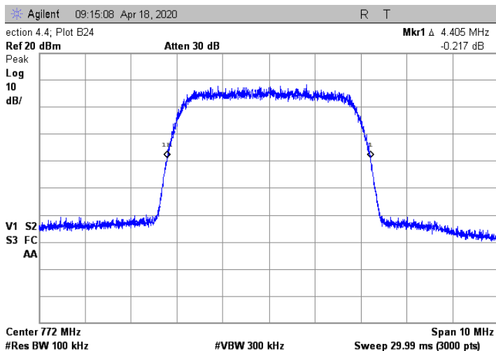
AMP Output, AWGN
