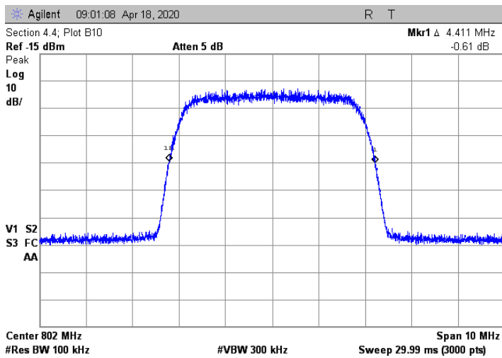
Generator; AWGN
