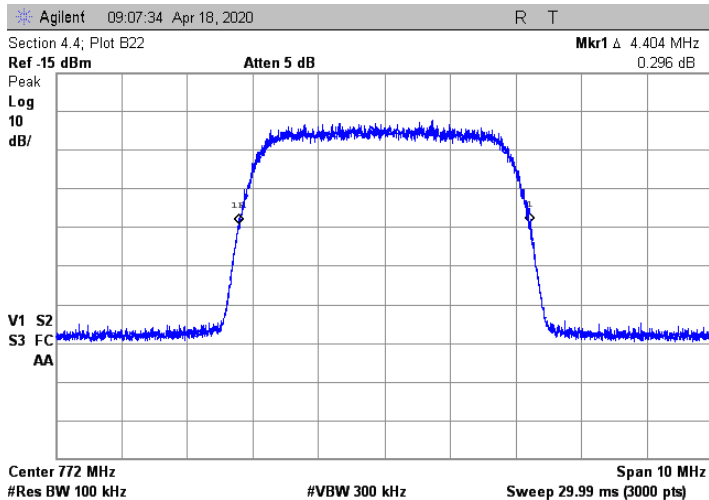
Generator; AWGN
