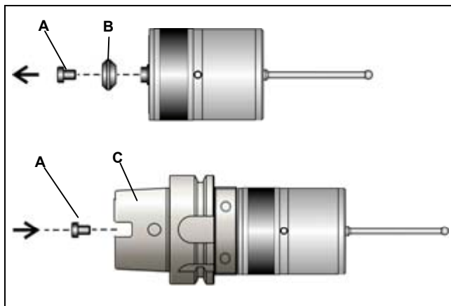
Figura 12-7. Fijación del transmisor al cono
