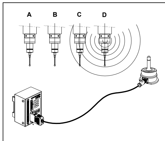
Abbildung 6-1. Funkübertragungssystem.
