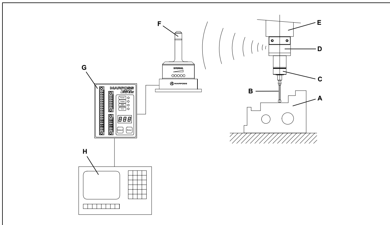
Figura 3-1. Configurazione e funzionamento.
