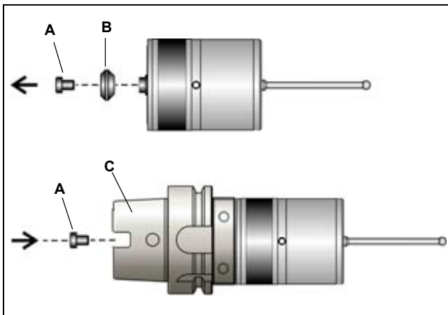
Abbildung 12-7. Befestigung des Sendermoduls am Kegel
