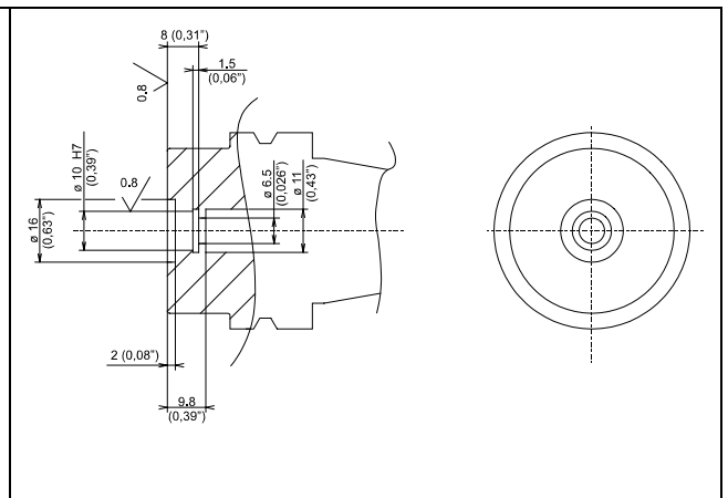
Abbildung 12-8. Bearbeitung des Kegels
