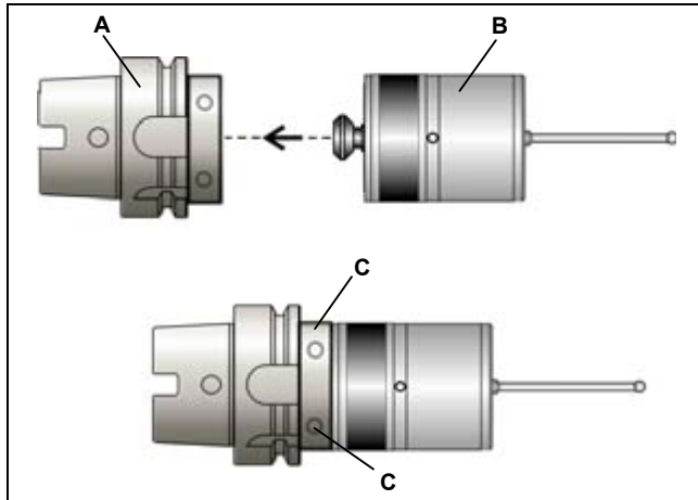
Figura 12-5. Fijación del transmisor al cono.
