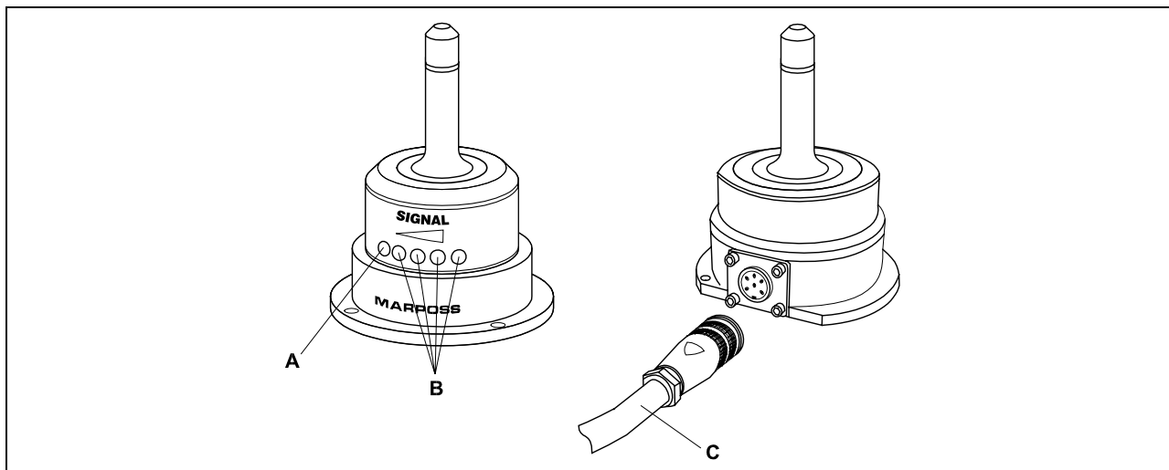
Figura 8-1: Antena y cable con conector.
