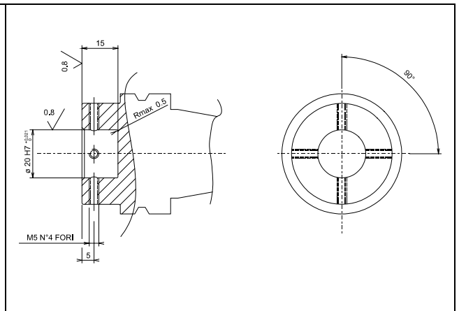
Figure 12-6. Percer le cône
