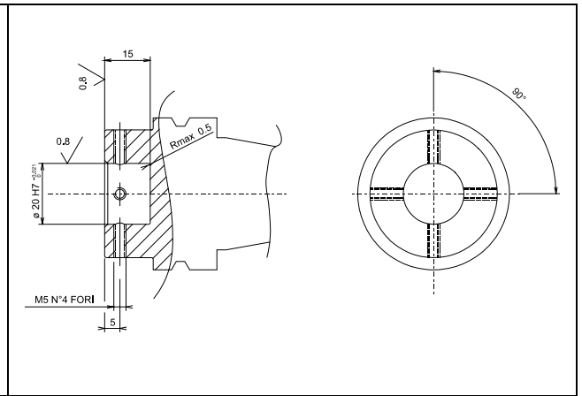
Abbildung 12-6. Bearbeitung des Kegels
