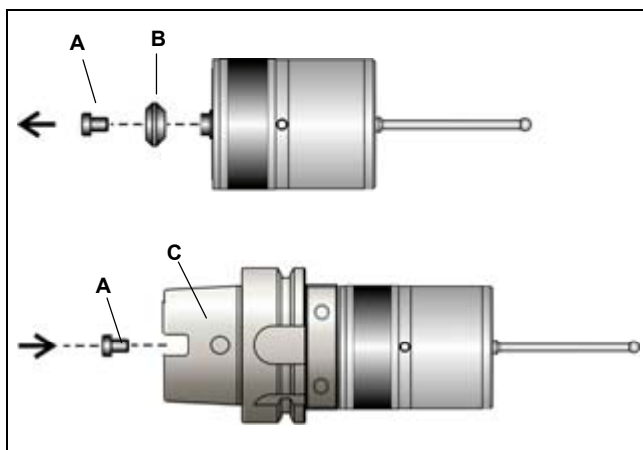
Figure 12-7. Fixer l'émetteur sur le cône
