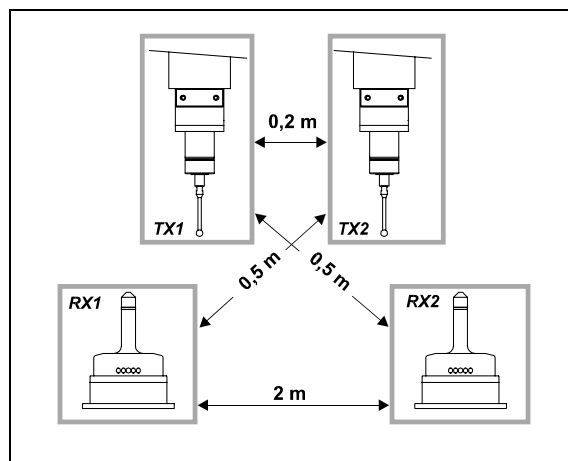
Abbildung 6-2. Abstand bei Verwendung von mehreren Systemen
