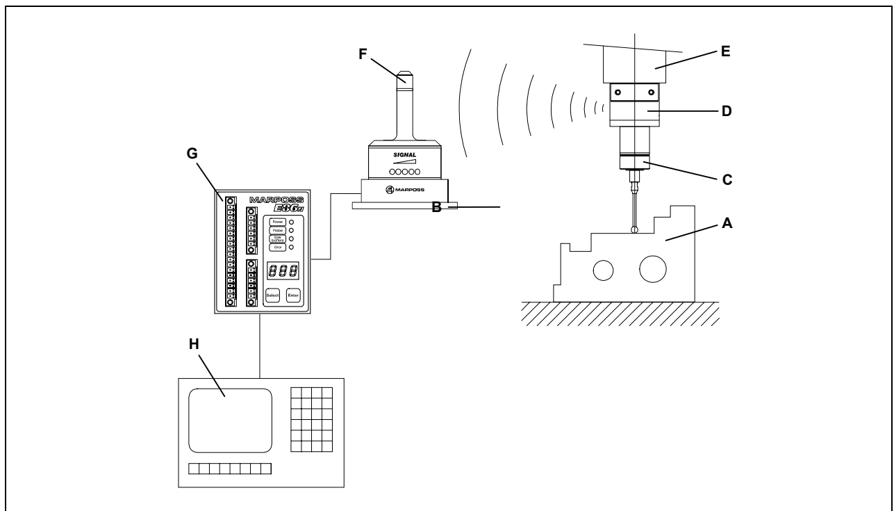
Figure 3-1. Configuration et fonctionnement
