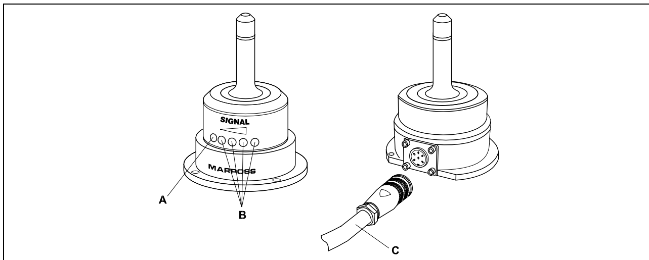
Abbildung 8-1: Empfängermodul mit steckbarem Anschlusskabel.
