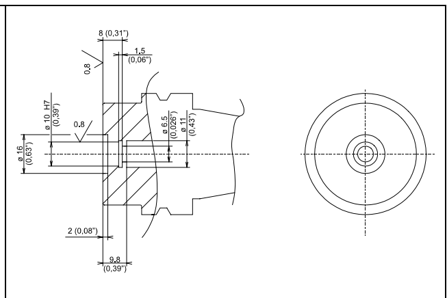
Figura 12-8. Mecanizado del cono.
