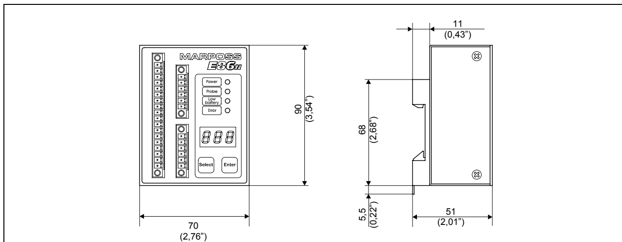
Figure 9-2. Dimensions hors tout
