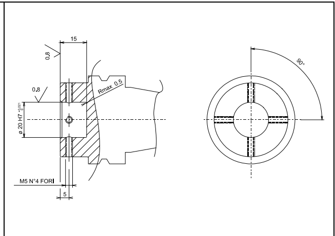
Figura 12-6. Mecanizado del cono.
