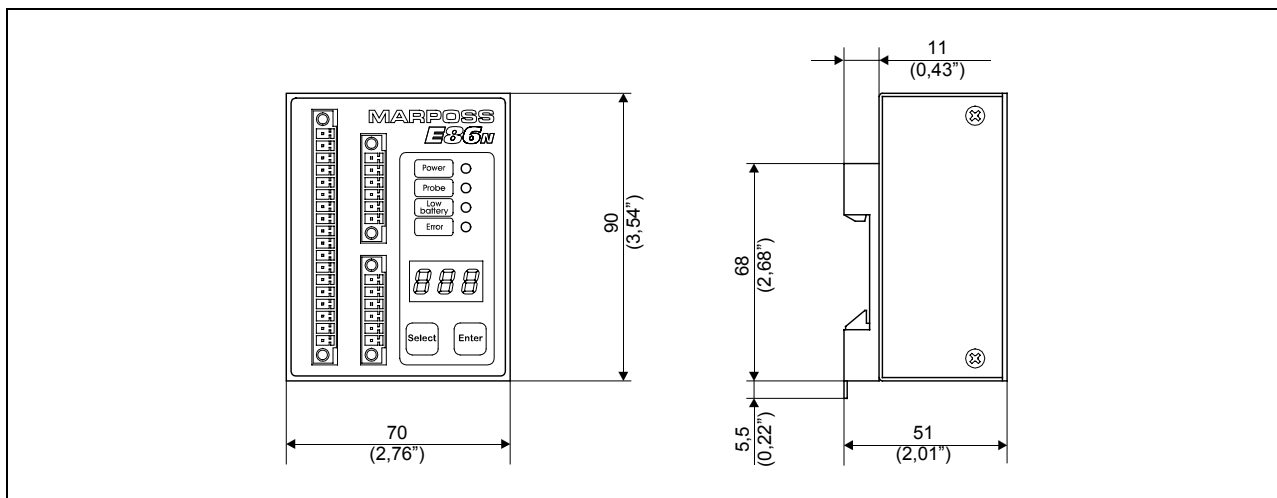
Figura 9-2. Dimensiones.
