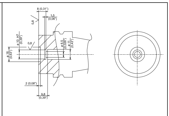
Figure 12-8. Percer le cône
