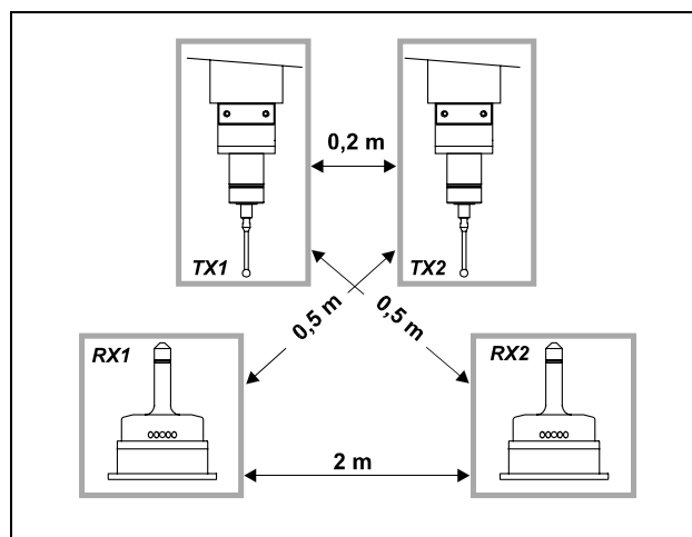
Figure 6-2. Distances mini entre systèmes
