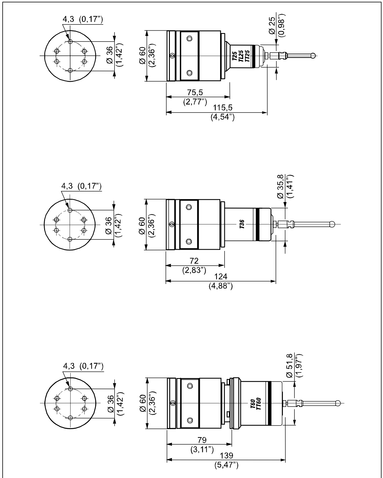
Abbildung 7-3. Abmessungen des Sendermoduls mit Regulierflansch.
