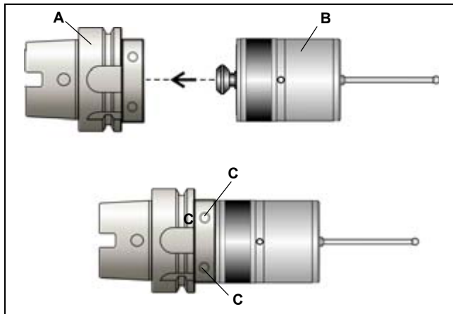
Figure 12-5. Fixer l'émetteur sur le cône
