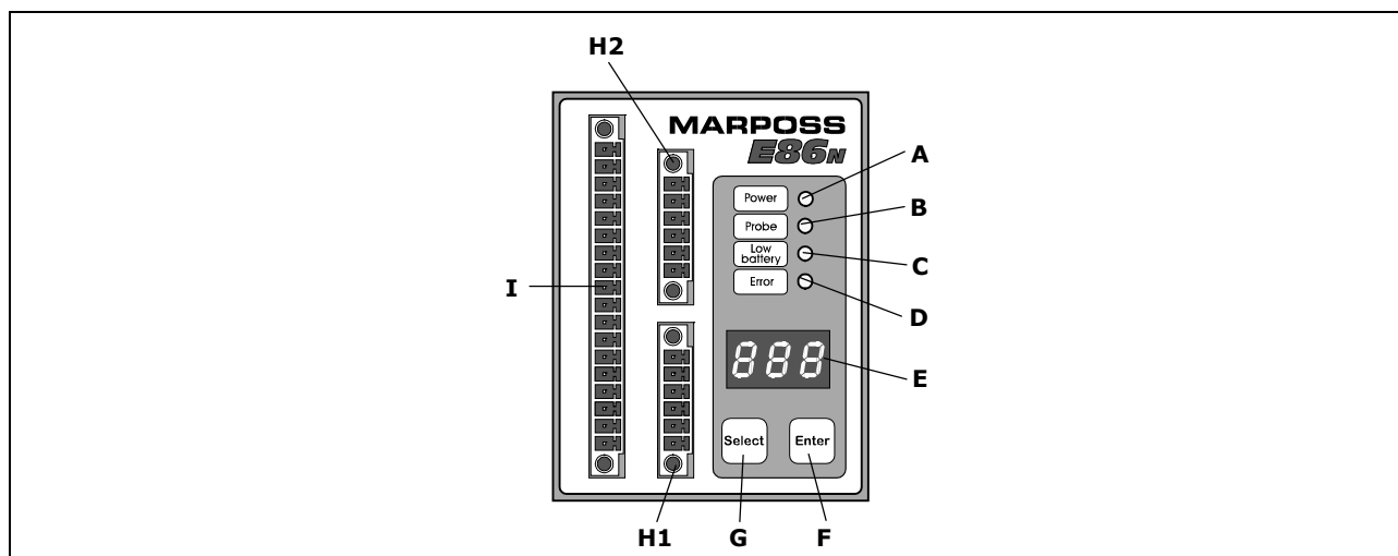
Figura9-1: Pannello frontale.
