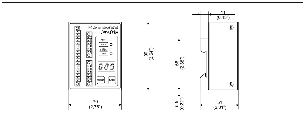
Abbildung 9-2. Abmessungen.
