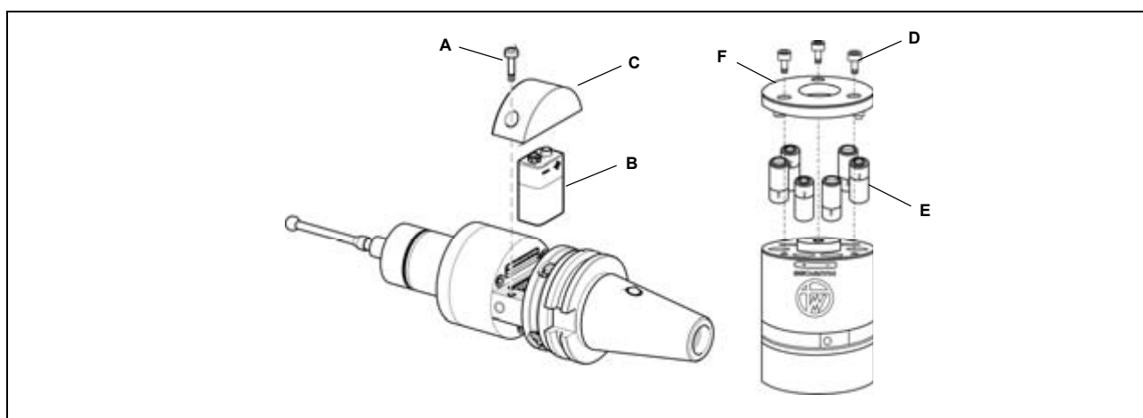
Abbildung 15-1. Einsetzen/Auswechseln der Batterien
