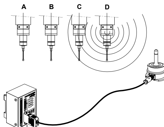
Figure 6-1. Système de transmission radio
