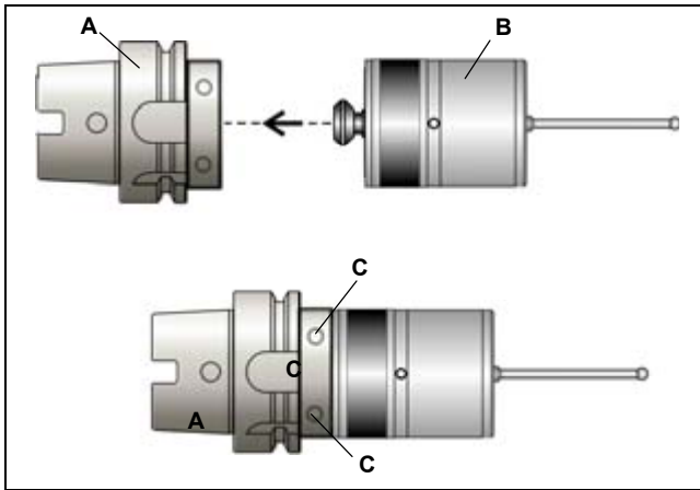
Abbildung 12-5. Befestigung des Sendermoduls am Kegel.
