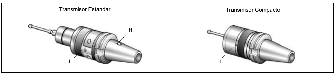
Figura 7-1. Transmisores.
