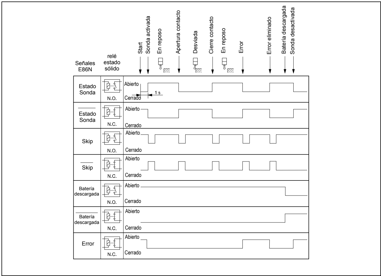
Figura 9-4. Diagrama I/O unidad de Interfaz.
