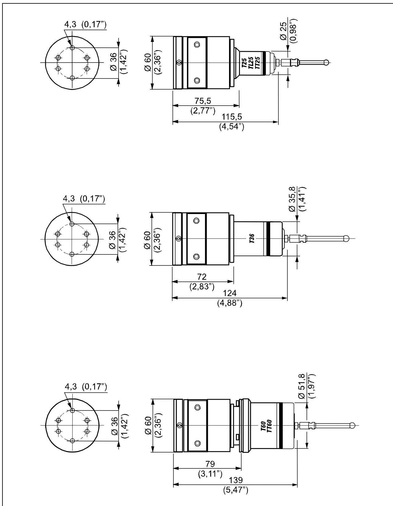
Figura 7-3. Ingombri trasmettitore con flangia di regolazione.
