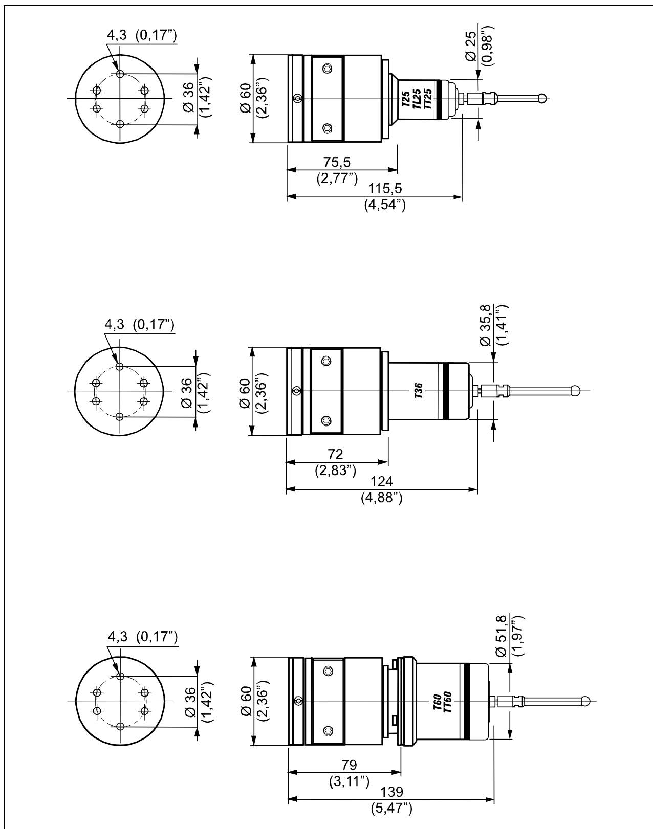
Figura 7-3. Dimensiones transmisor con brida de regulación.
