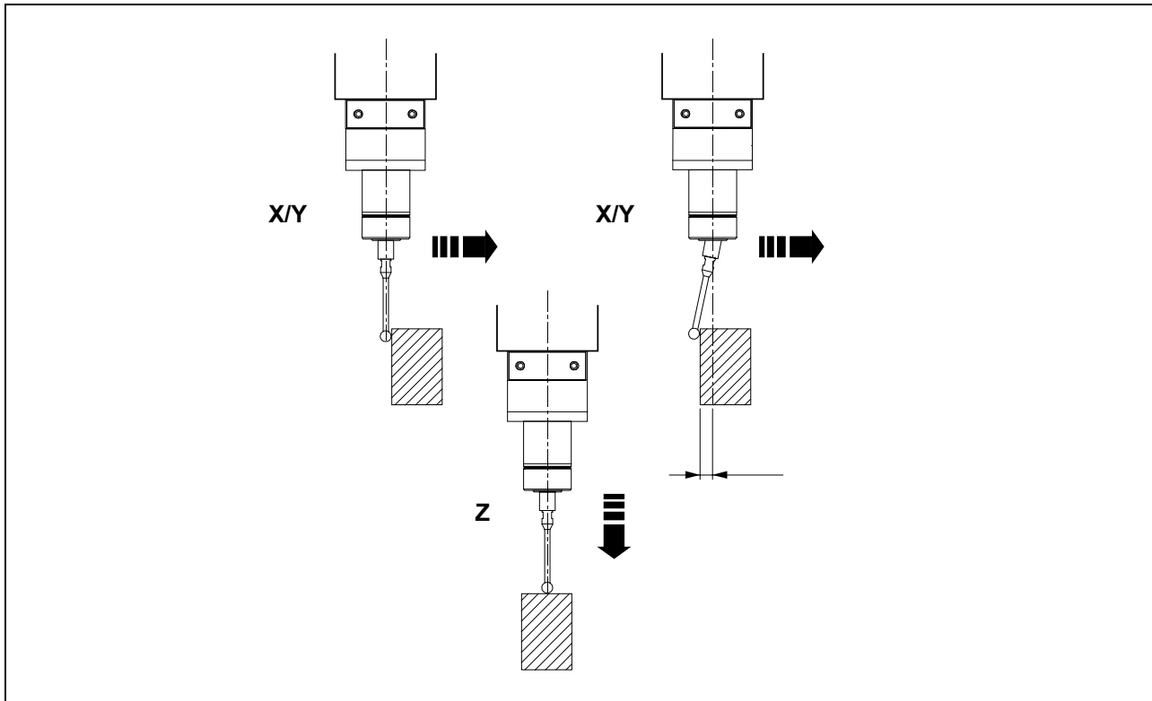
Figura 4-1. Modalità d'impiego.
