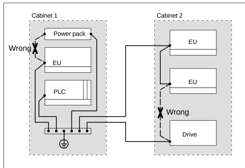
Figure 3-8 Equipotential bonding
