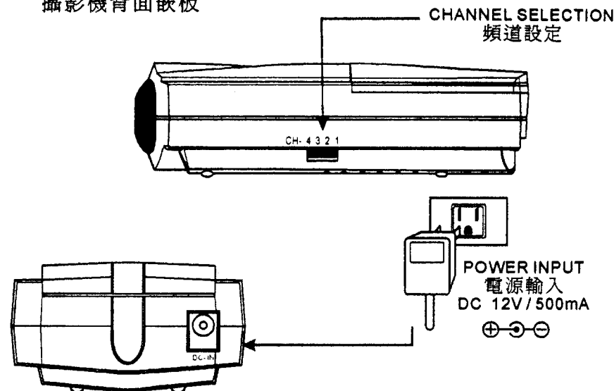
Video Camera Back Panel 攝影機背面嵌板
