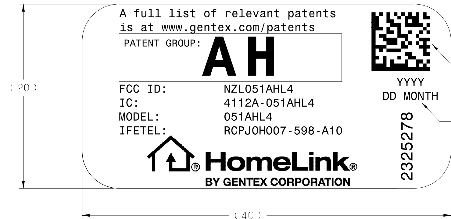
LABEL VIEW SCALE: 4:1
