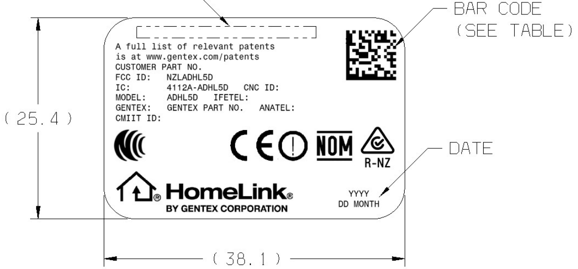
PATENT LABEL 'M' - ITEM 2 SCALE: 2:1
