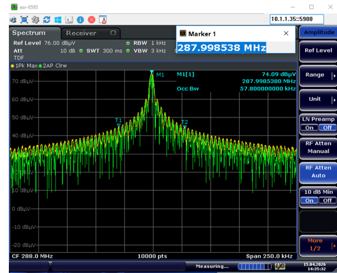
99% BW
