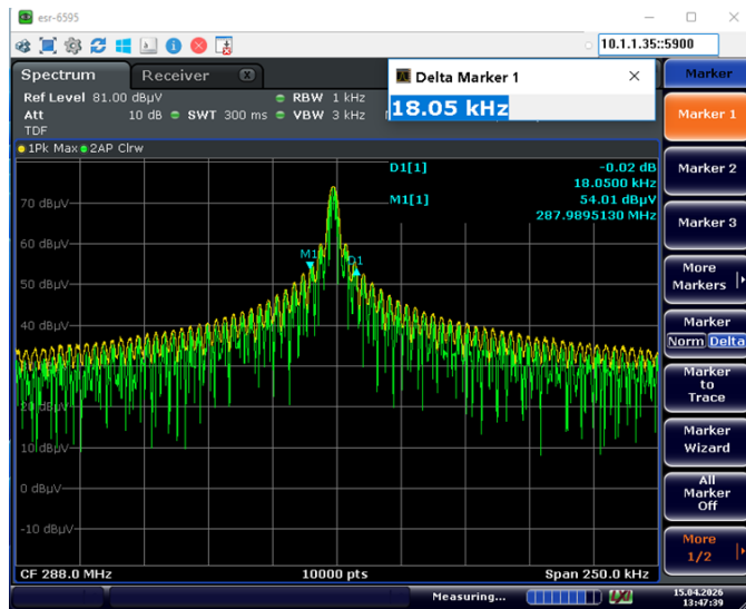
20dB BW
