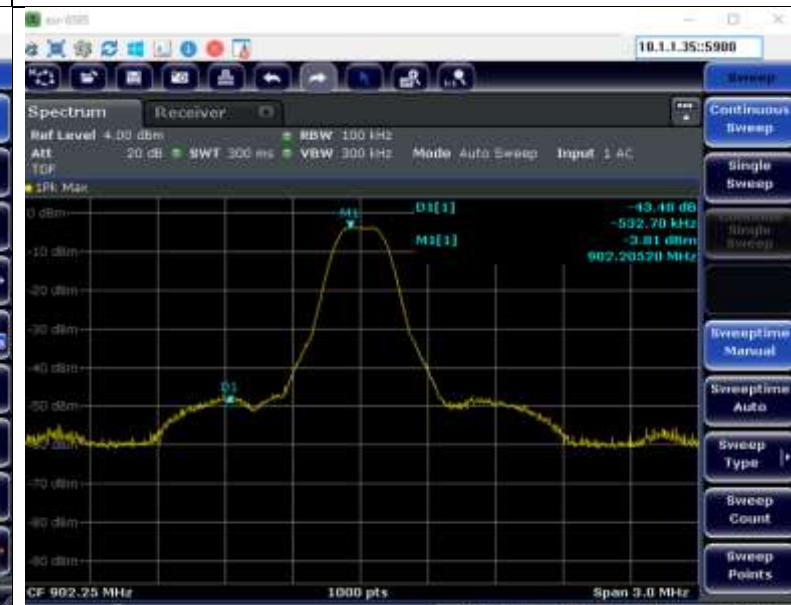
Non - Hopping Low Frequency Band Edge
