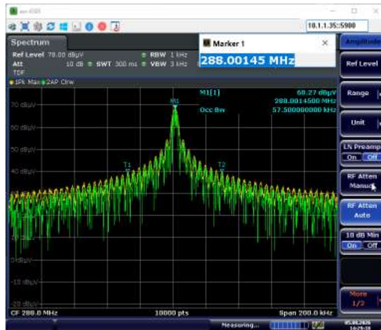
20dB BW
