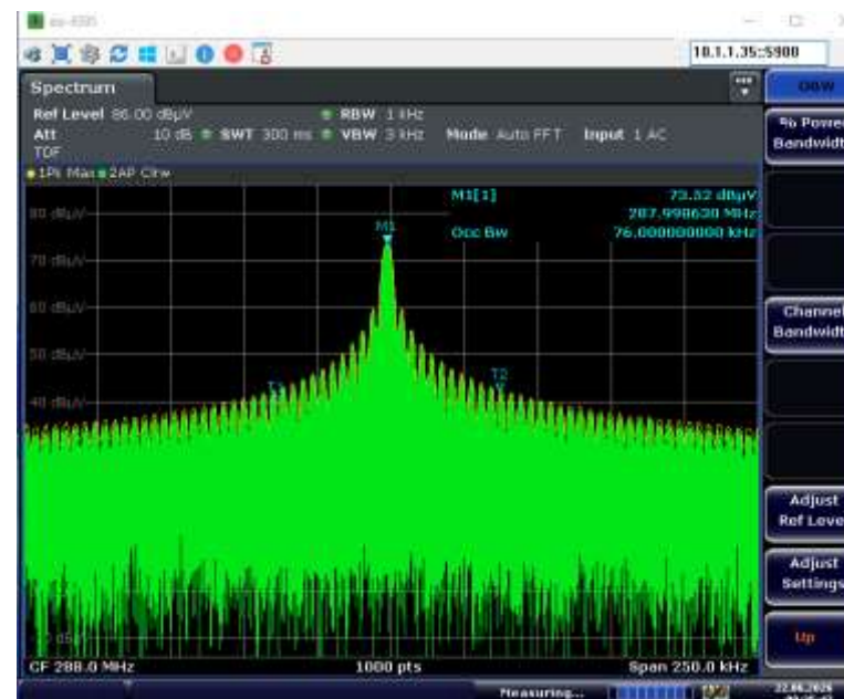
99% BW
