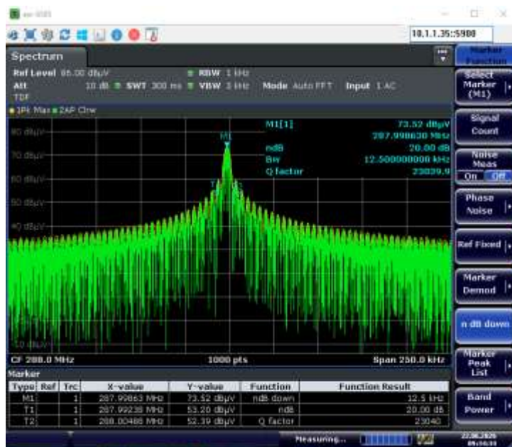
20dB BW
