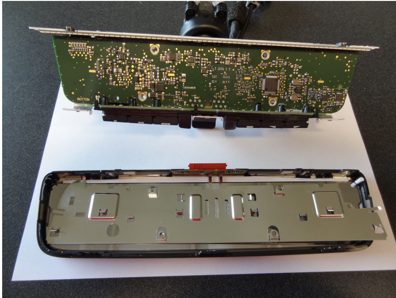
UAHL5E – Internal Photos
