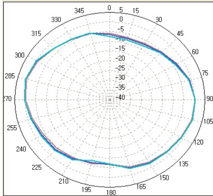
E2 plan
