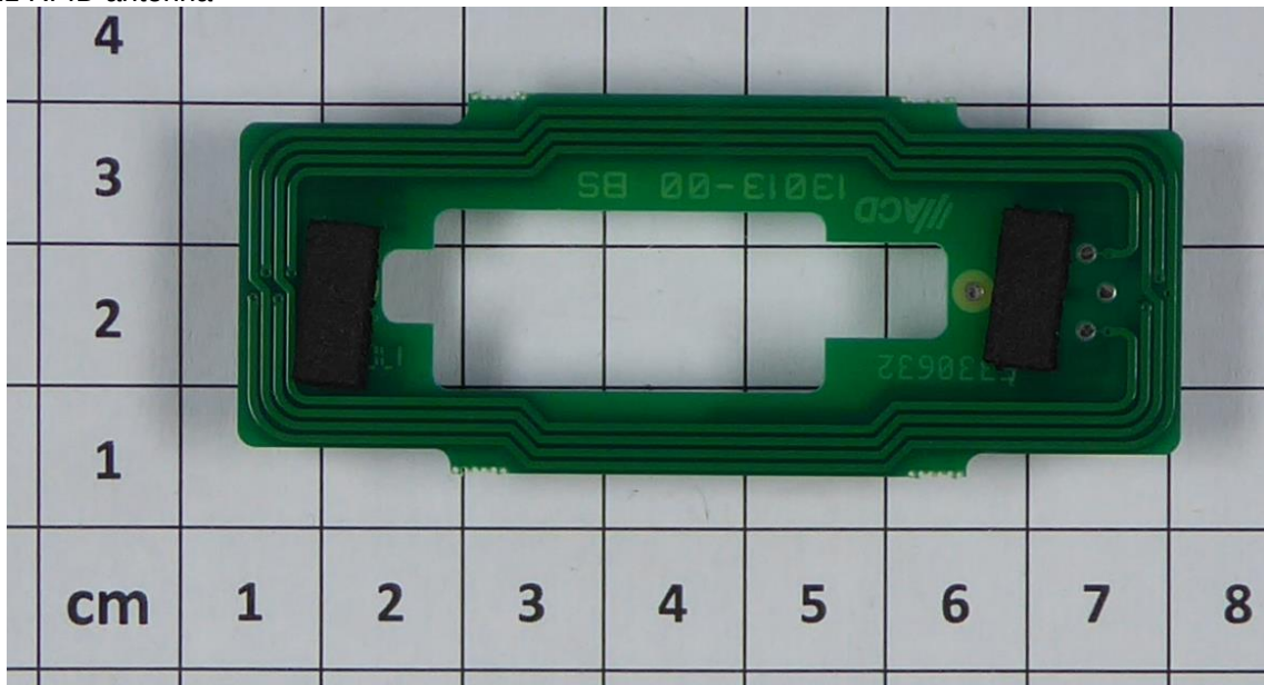
13.56 MHz RFID antenna
