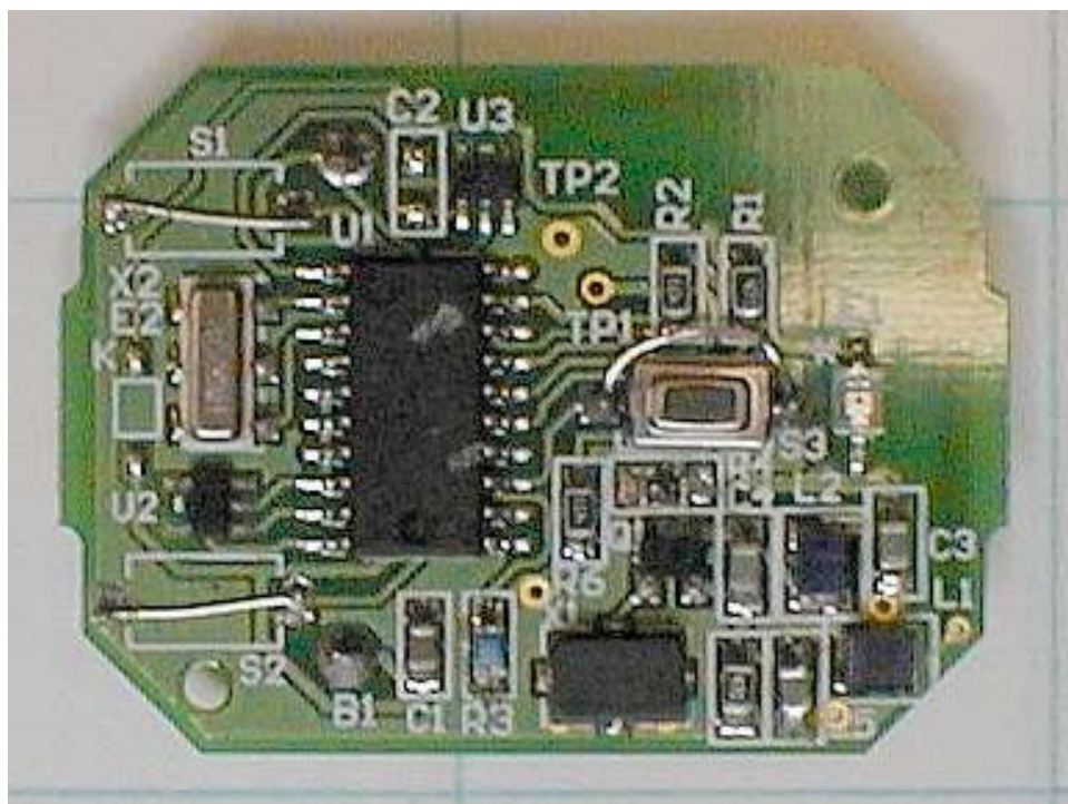
PCB Top
