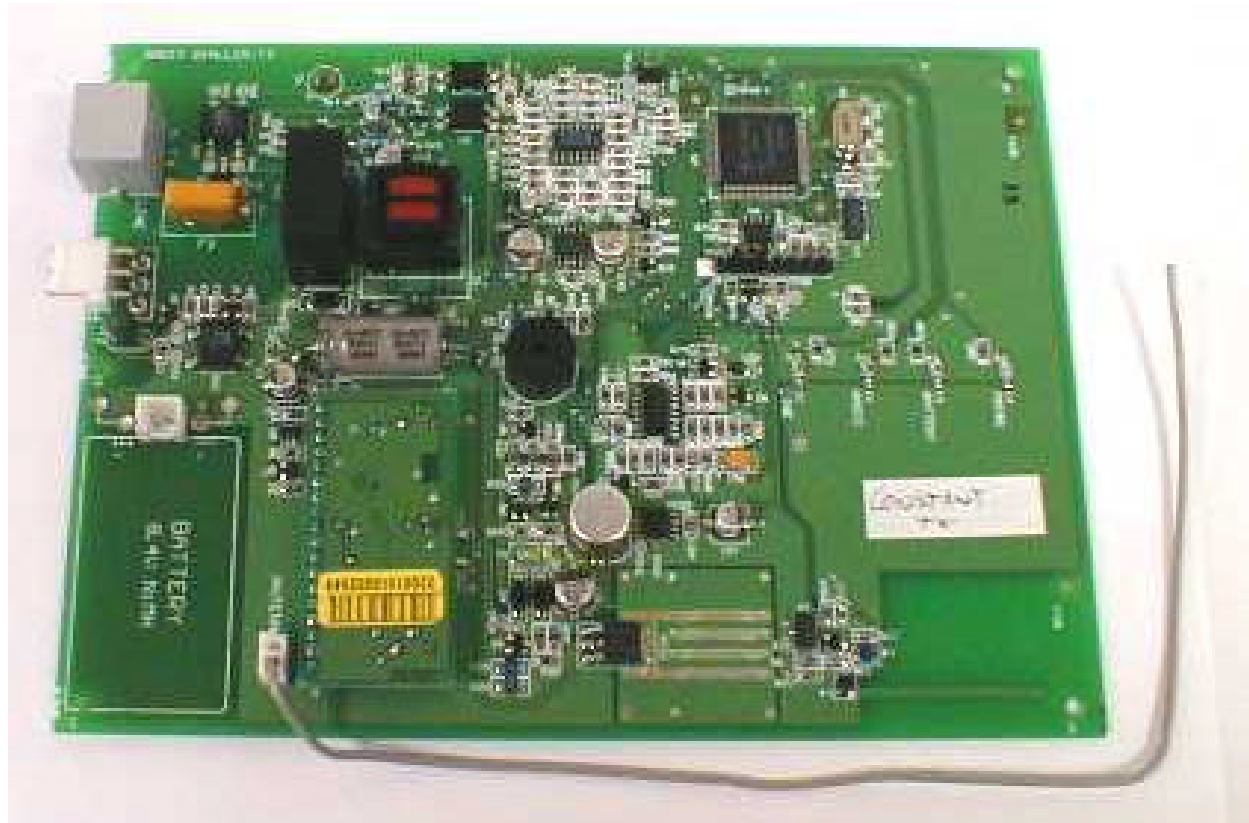
PCB Top
