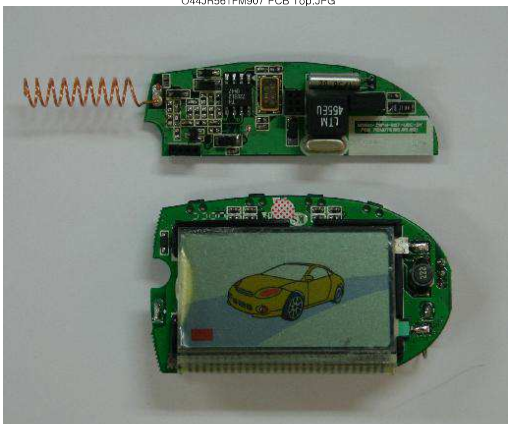
O44JR561FM907 PCB Top.JPG
