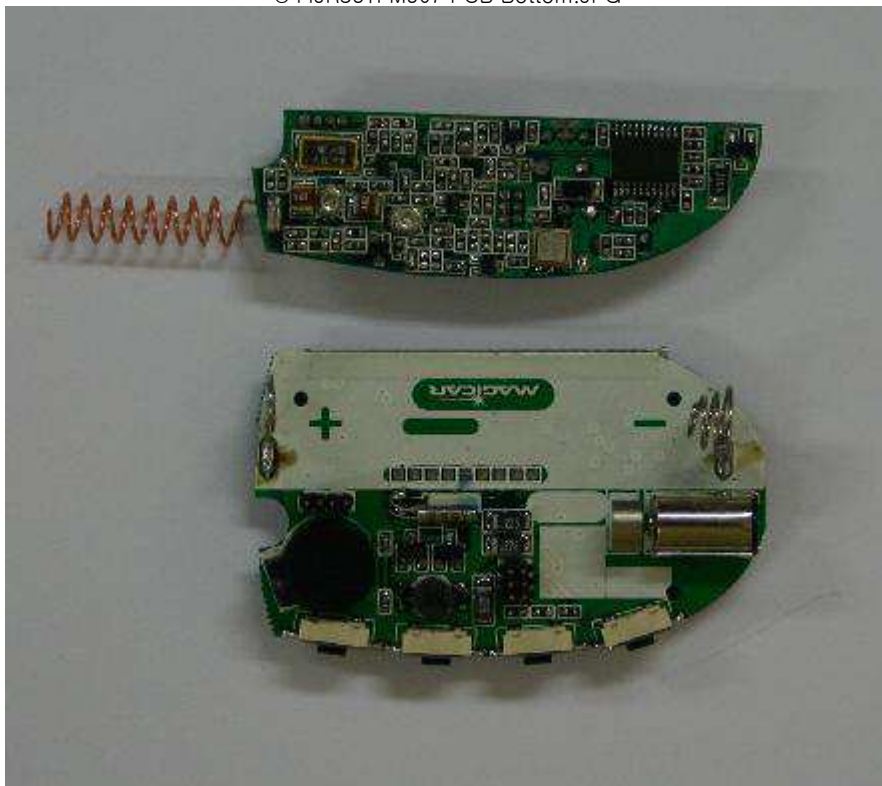
O44JR561FM907 PCB Bottom.JPG
